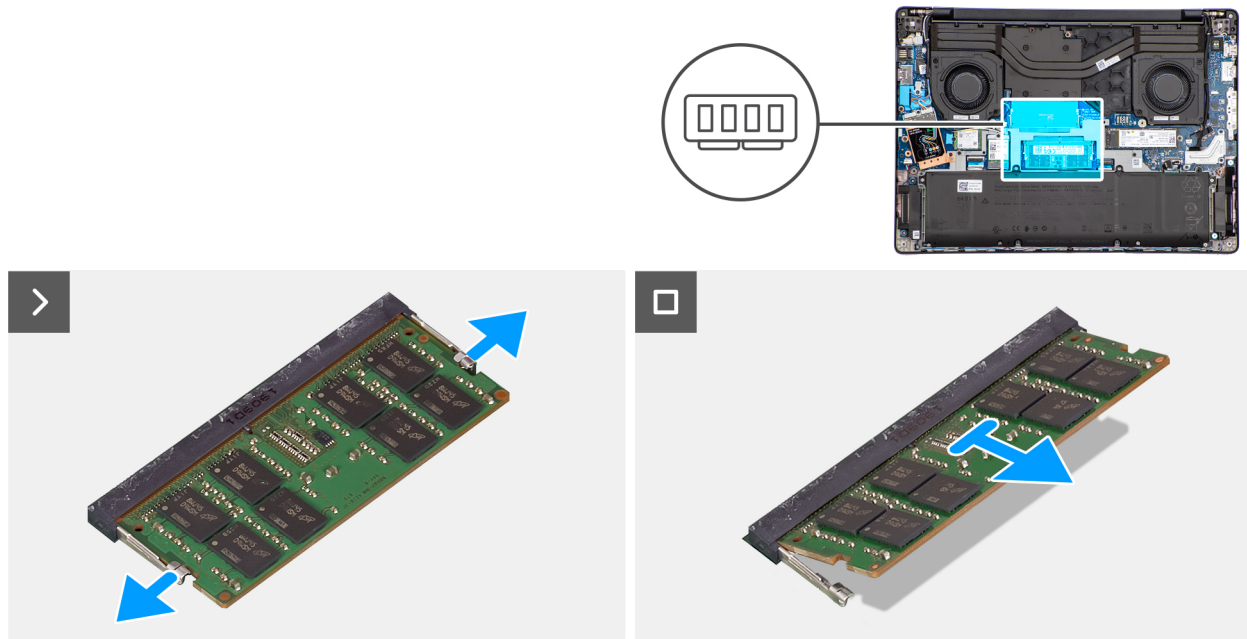
Abbildung 21. Entfernen des Arbeitsspeichermoduls
