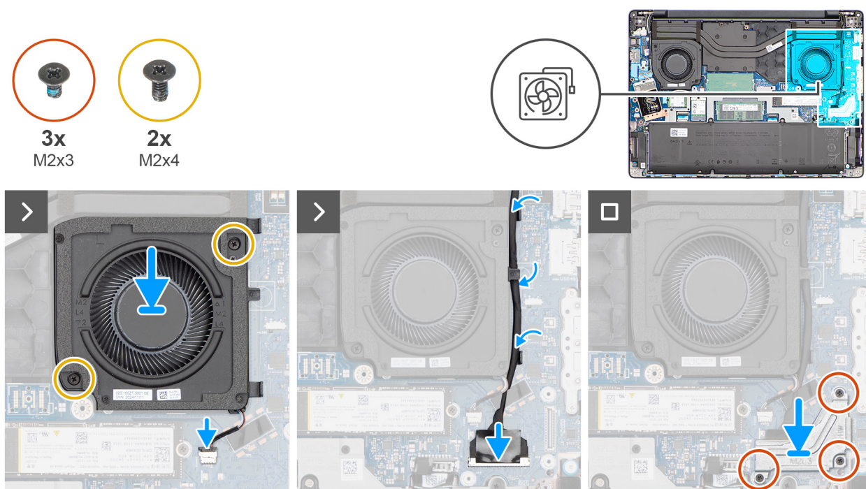
Abbildung 39. Einbauen des linken/Videolüfters
