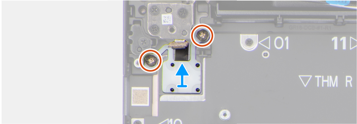
Abbildung 96. Entfernen des Netzschalters
