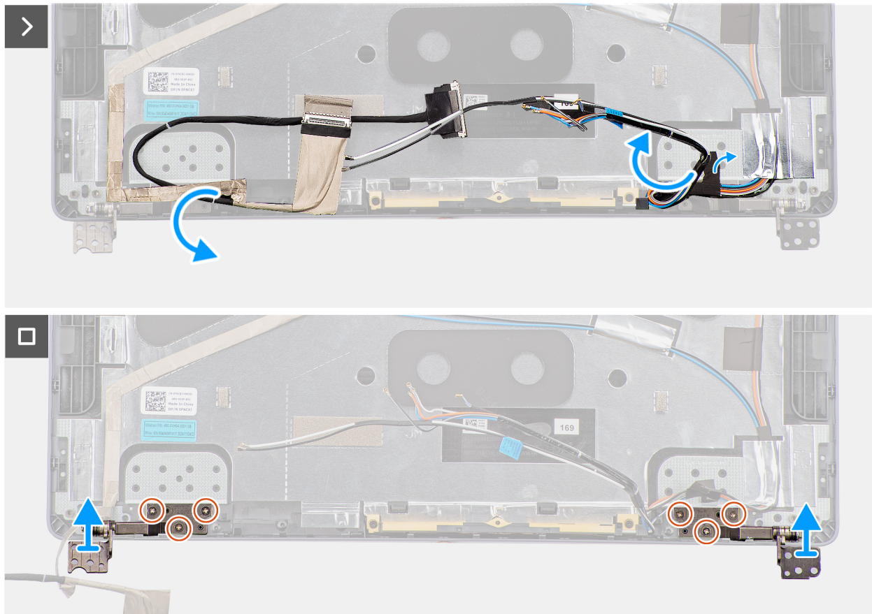
Abbildung 74. Entfernen der Bildschirmscharniere
