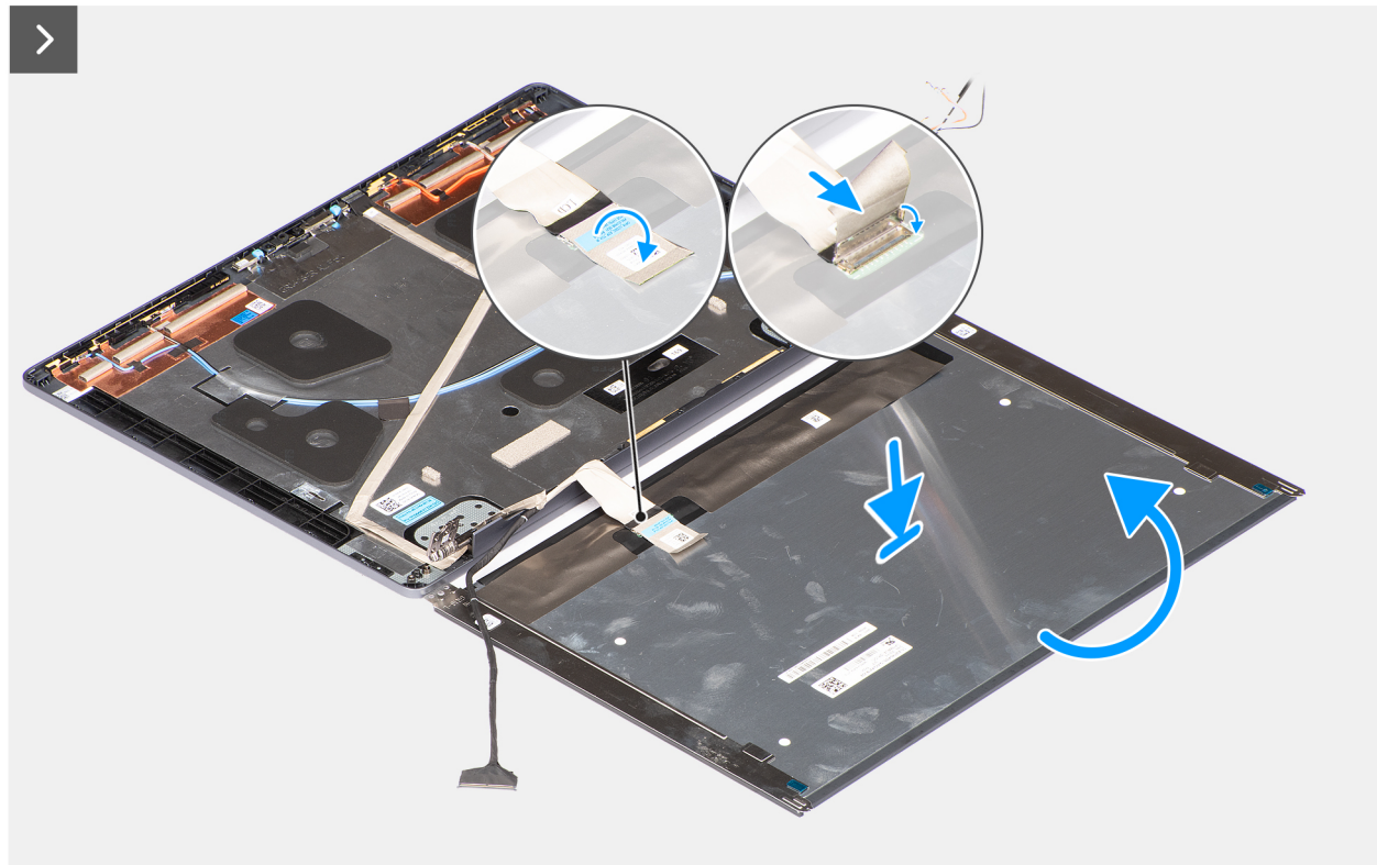
Abbildung 72. Einbauen des Bildschirms
