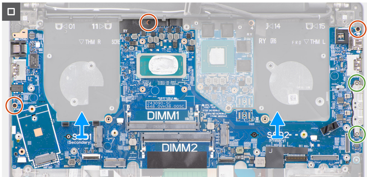
Abbildung 90. Entfernen der Systemplatine
