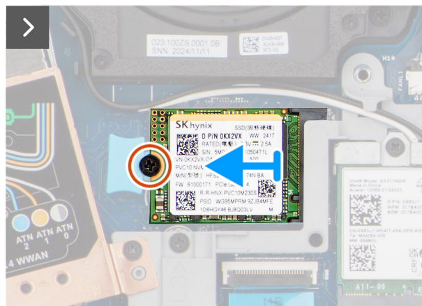
Abbildung 23. Entfernen des M.2-2230-Solid-State-Laufwerks
