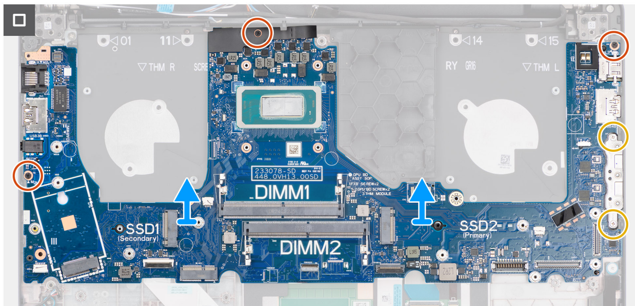
Abbildung 84. Entfernen der Systemplatine
