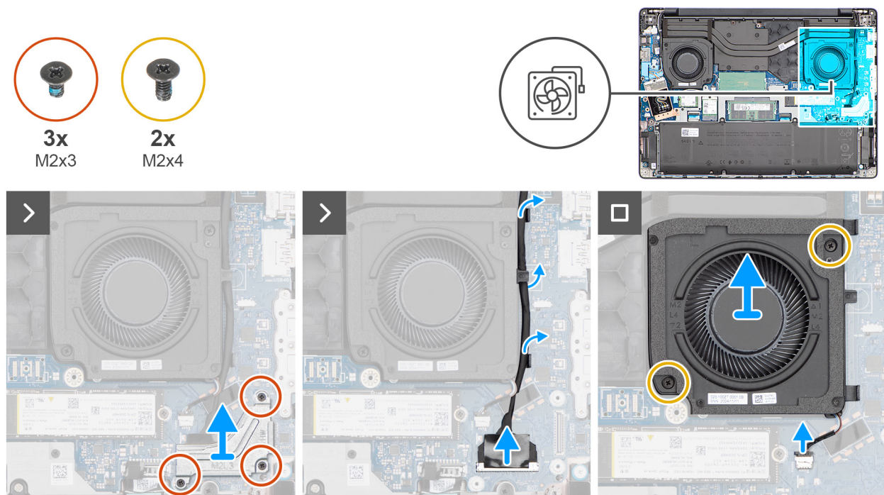
Abbildung 38. Entfernen des linken/Videolüfters
