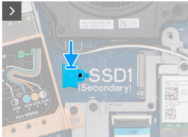
Abbildung 24. Installieren des M.2 2230-Solid-State-Laufwerks
