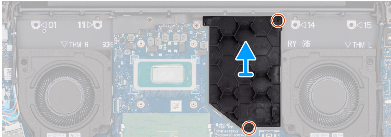
Abbildung 44. Entfernen des GPU-Platzhalters
