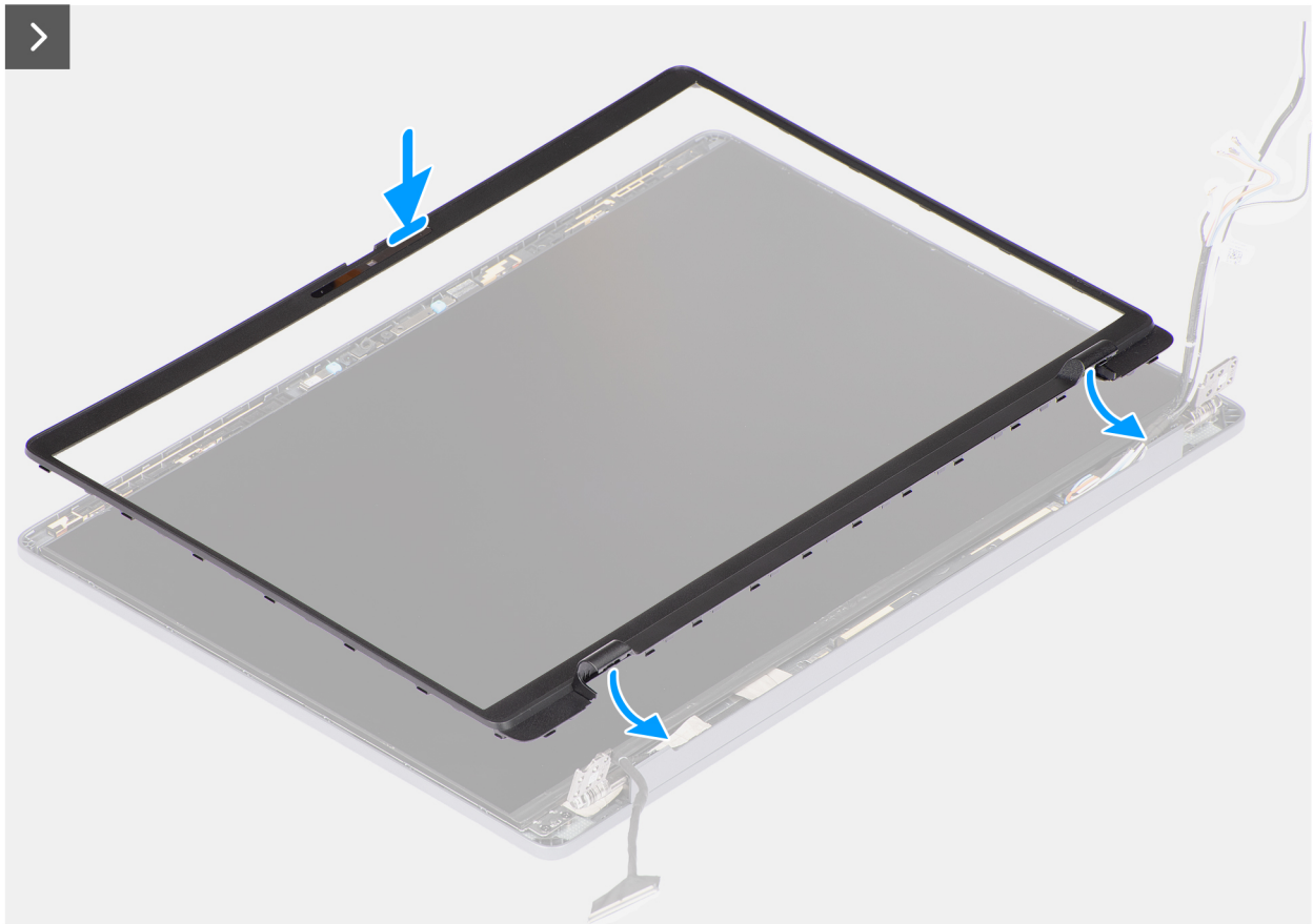
Abbildung 66. Einbauen der Bildschirmblende
