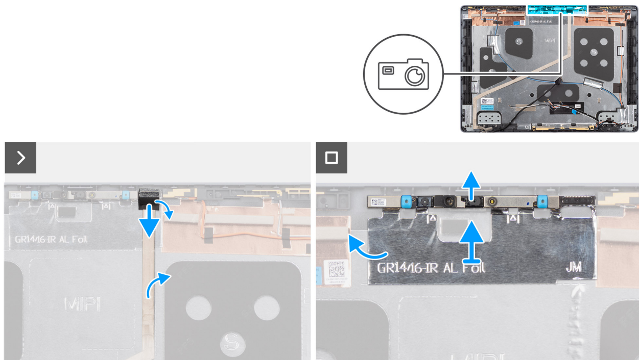
Abbildung 78. Entfernen der Kamera
