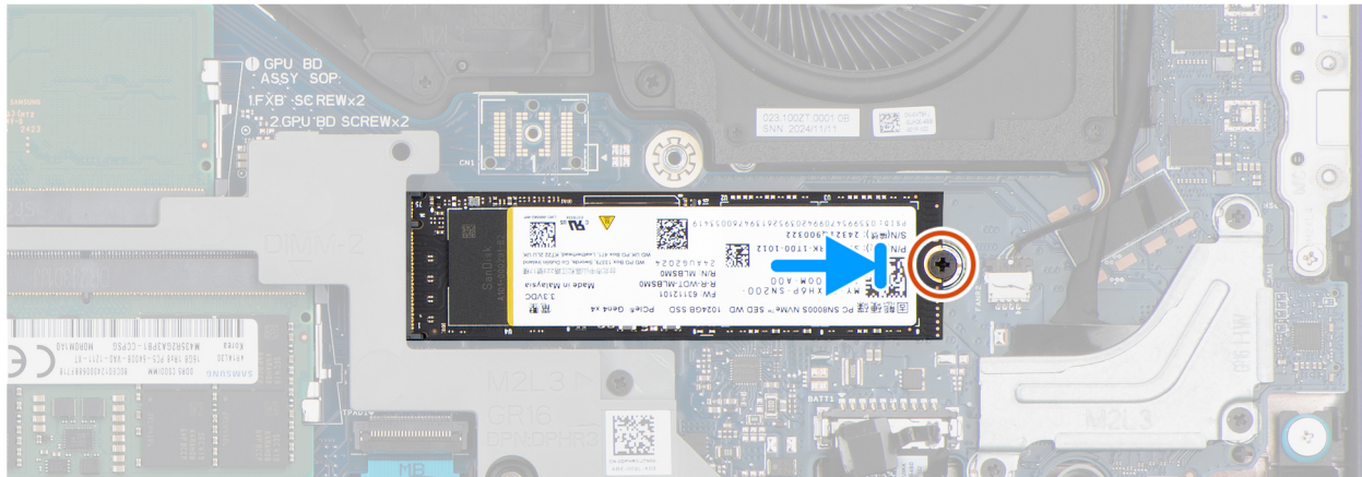
Abbildung 26. Installieren des M.2 2280-Solid-State-Laufwerks
