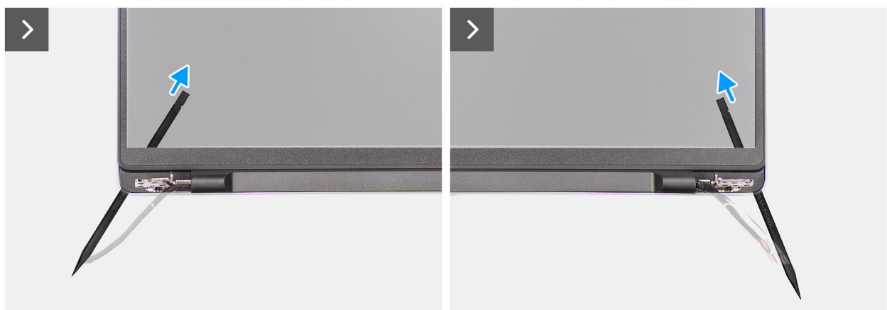
Abbildung 61. Entfernen der Bildschirmblende
