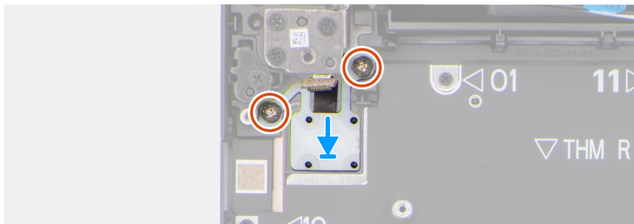
Abbildung 97. Installieren des Netzschalters
