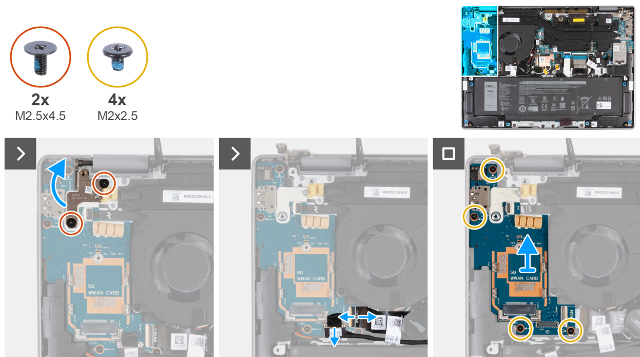
Abbildung 85. Entfernen der I/O-Platine (Computer mit WWAN-Unterstützung)
