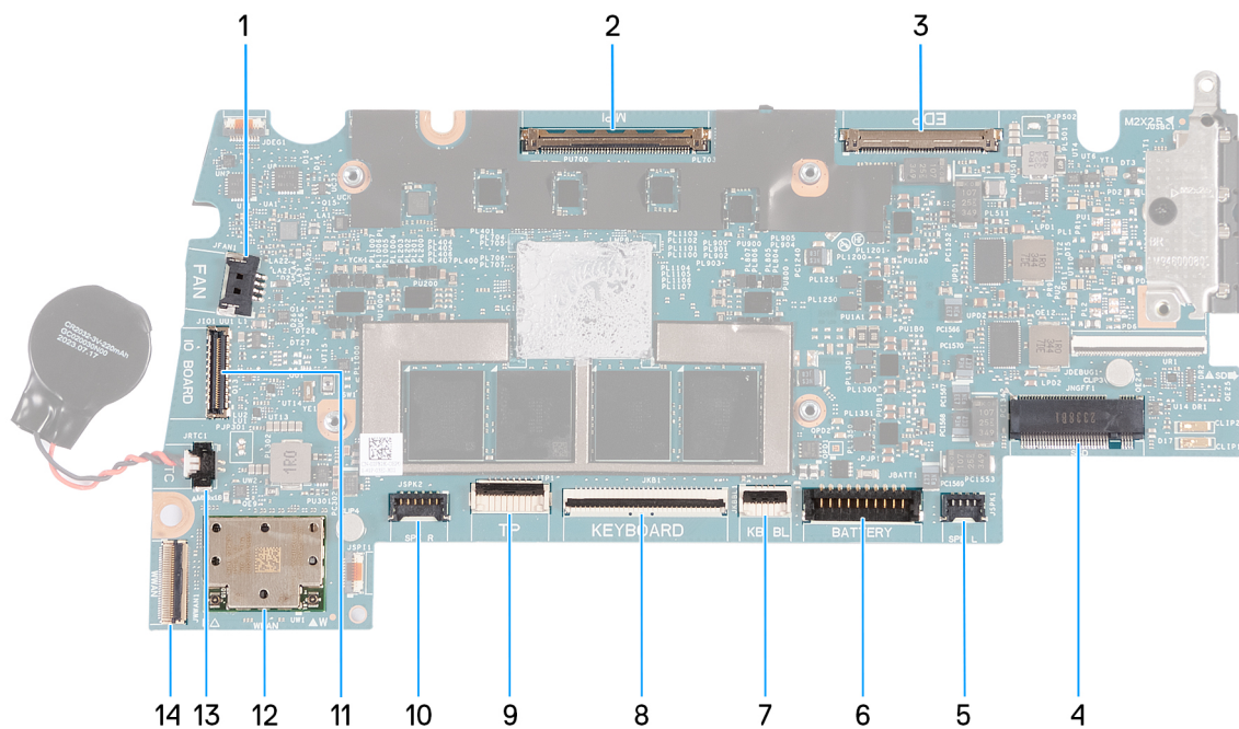
Abbildung 98. Hauptplattenanschlüsse
