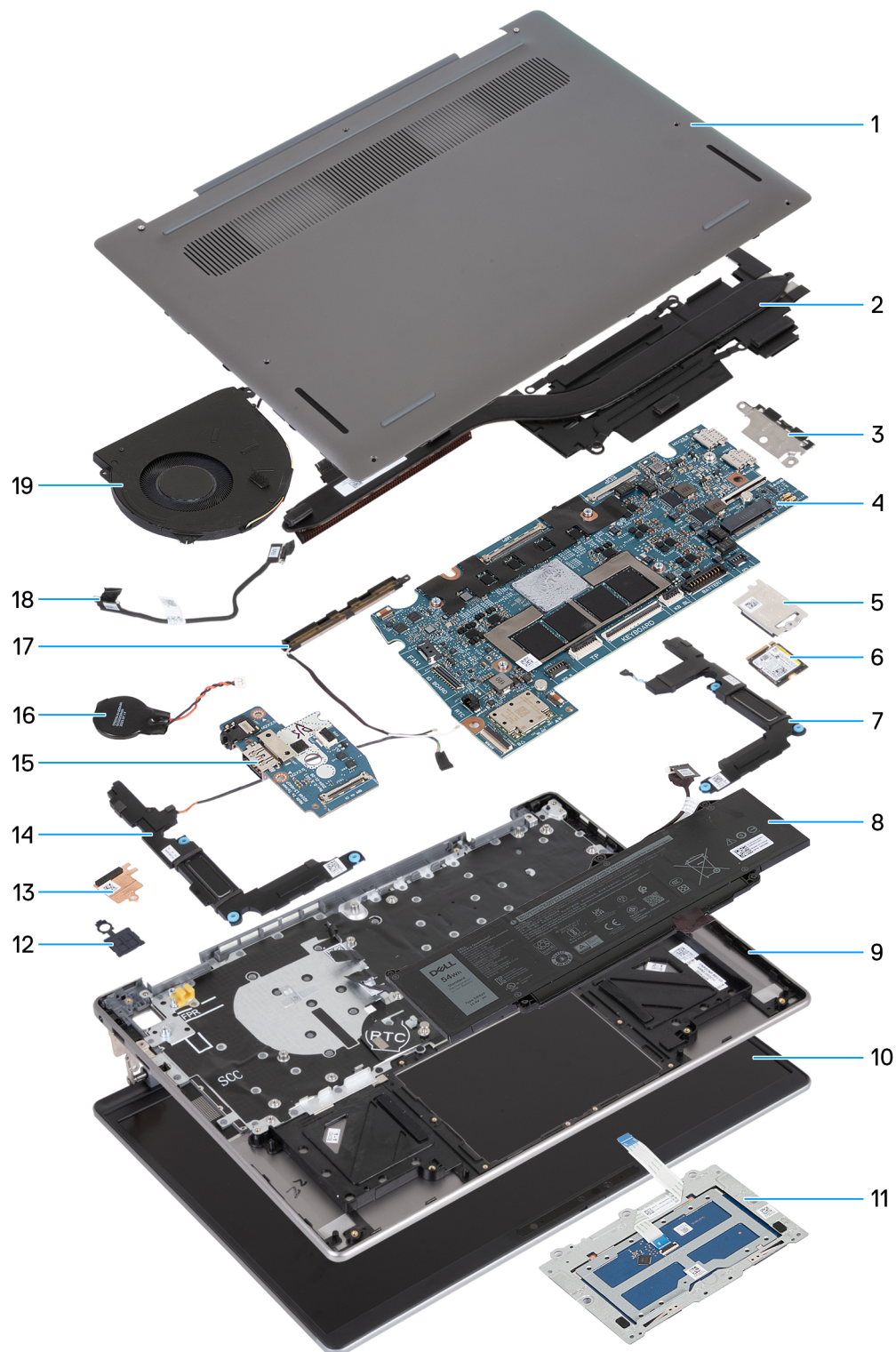
Abbildung 10. Hauptkomponenten des Latitude 7455 (bei Computern nur mit WLAN-Unterstützung)
