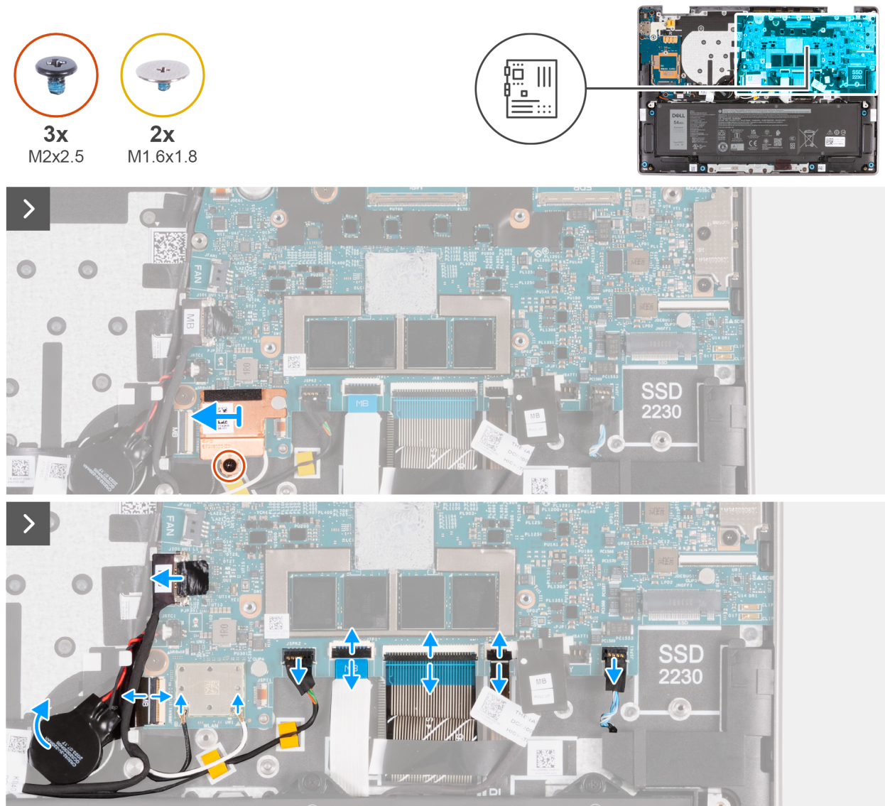
Abbildung 95. Entfernen der Systemplatine
