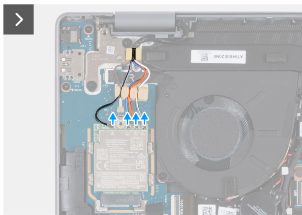
Abbildung 27. Entfernen der 5G-WWAN-Karte
