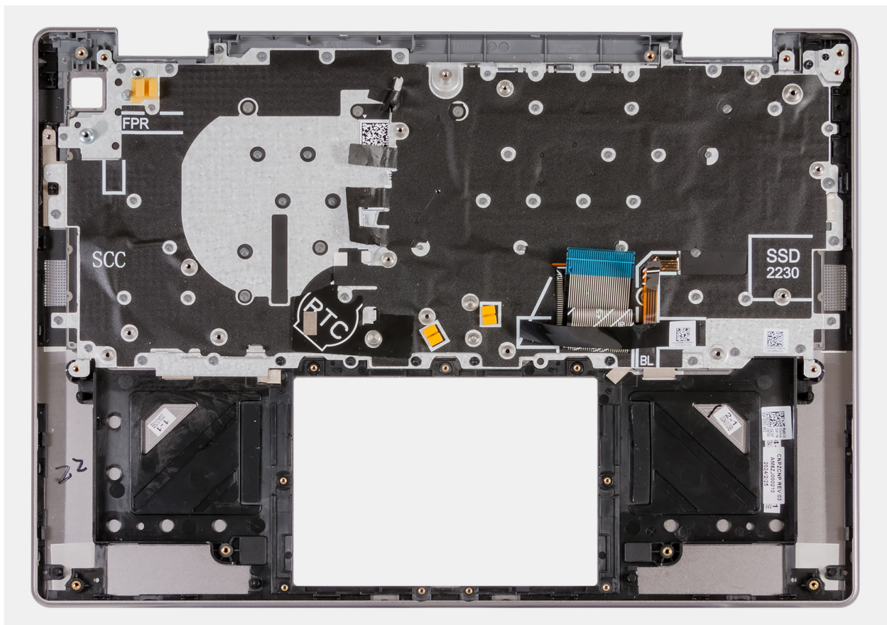
Abbildung 101. Handballenstützen- und Tastaturbaugruppe
