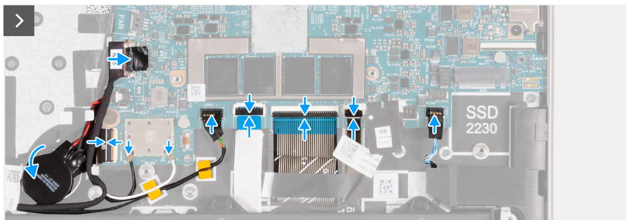
Abbildung 99. Einbauen der Systemplatine
