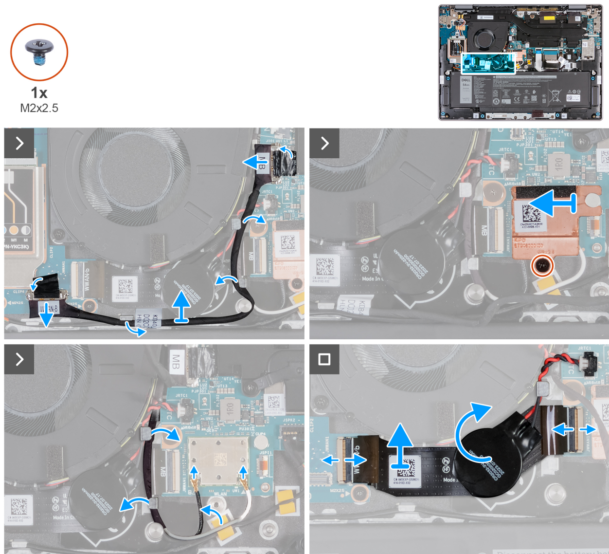
Abbildung 57. Entfernen des FPC-Kabels der I/O-Platine
