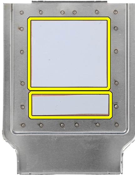
Abbildung 31. Wärmeleitpads an der Unterseite der WWAN-Kühlabdeckung
