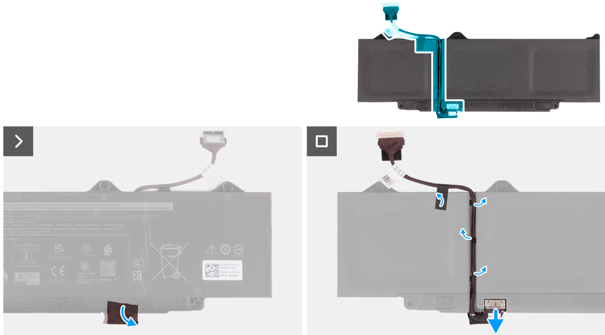
Abbildung 42. Entfernen des Akkukabels
