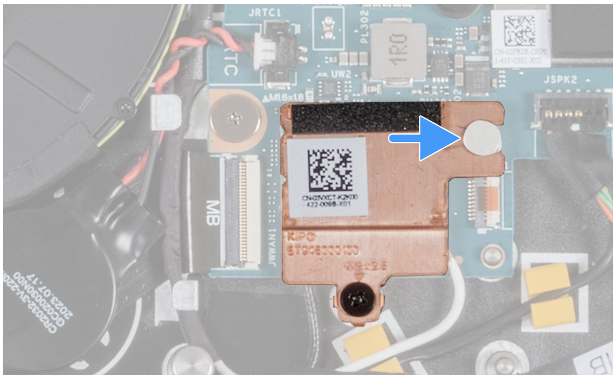
Abbildung 74. Installation der WLAN-Kühlabdeckung
