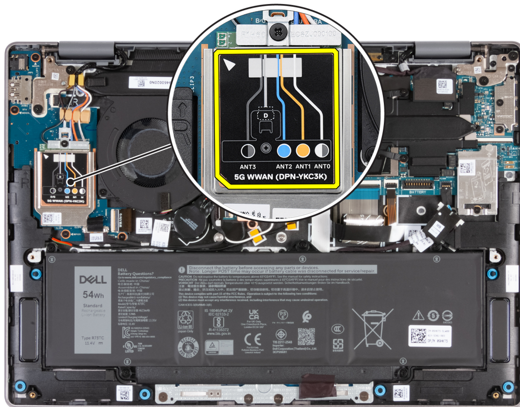
Abbildung 30. Antennenkabelverbindungen
