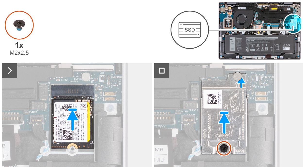
Abbildung 24. Einbauen der SSD
