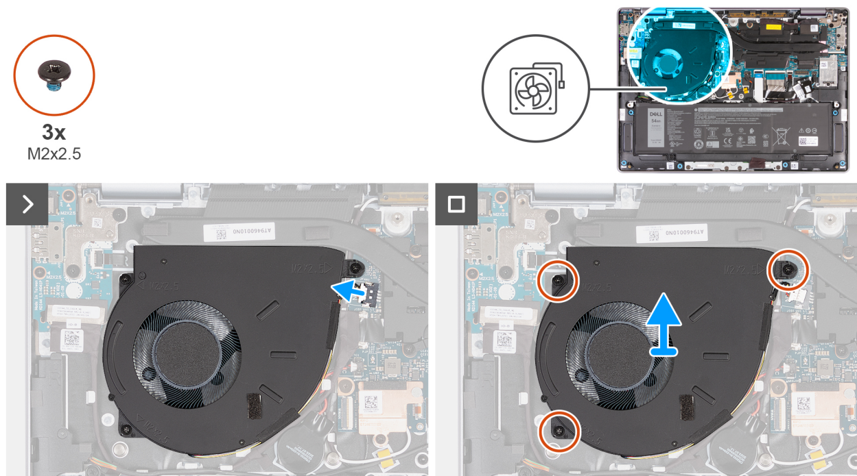
Abbildung 36. Entfernen des Lüfters (bei Computern nur mit WLAN-Unterstützung)
