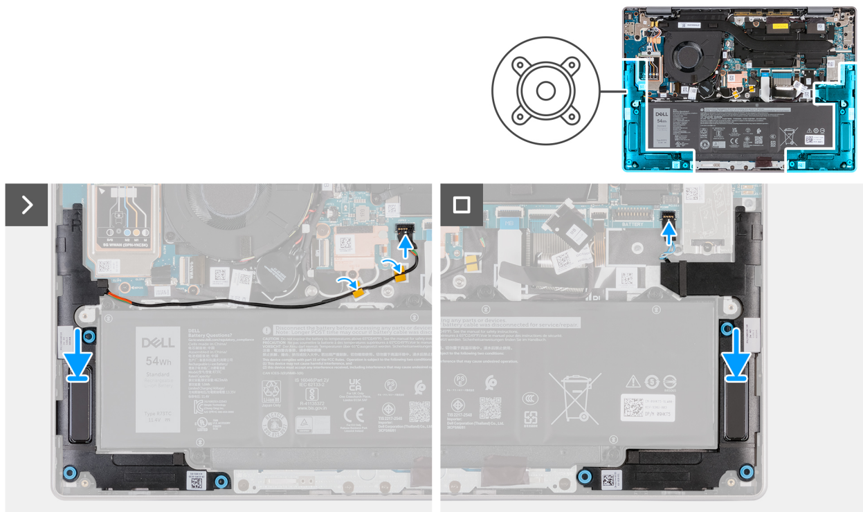
Abbildung 34. Einbauen der Lautsprecher
