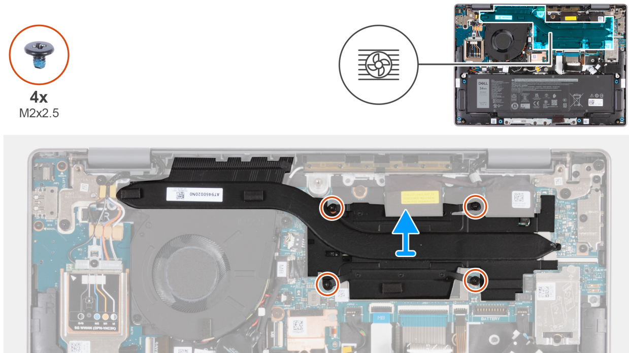
Abbildung 45. Entfernen des Kühlkörpers
