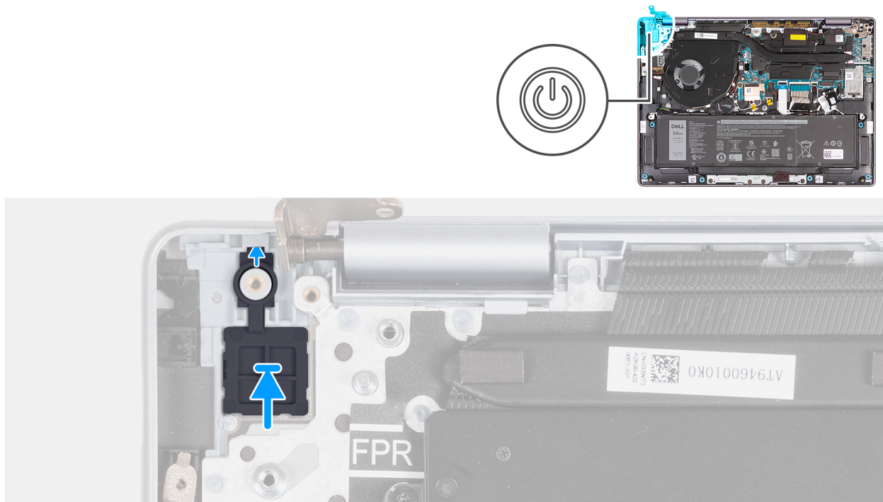
Abbildung 91. Einbauen des Netzschalters
