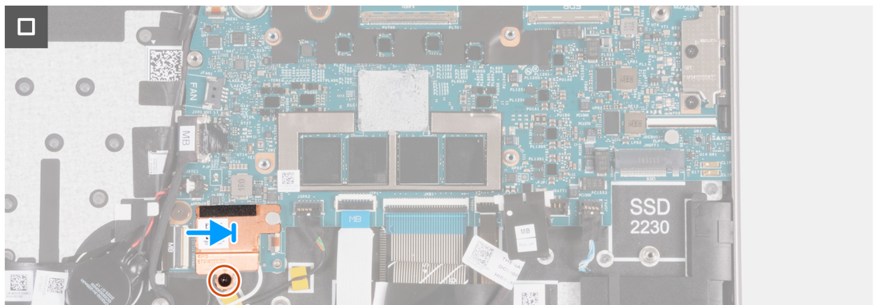
Abbildung 100. Einbauen der Systemplatine
