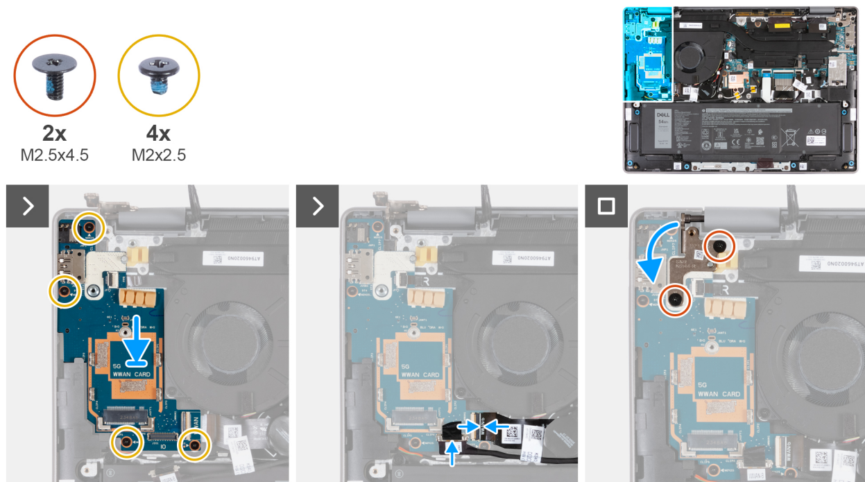
Abbildung 86. Installieren der I/O-Platine Entfernen der I/O-Platine (Computer mit WWAN-Unterstützung)
