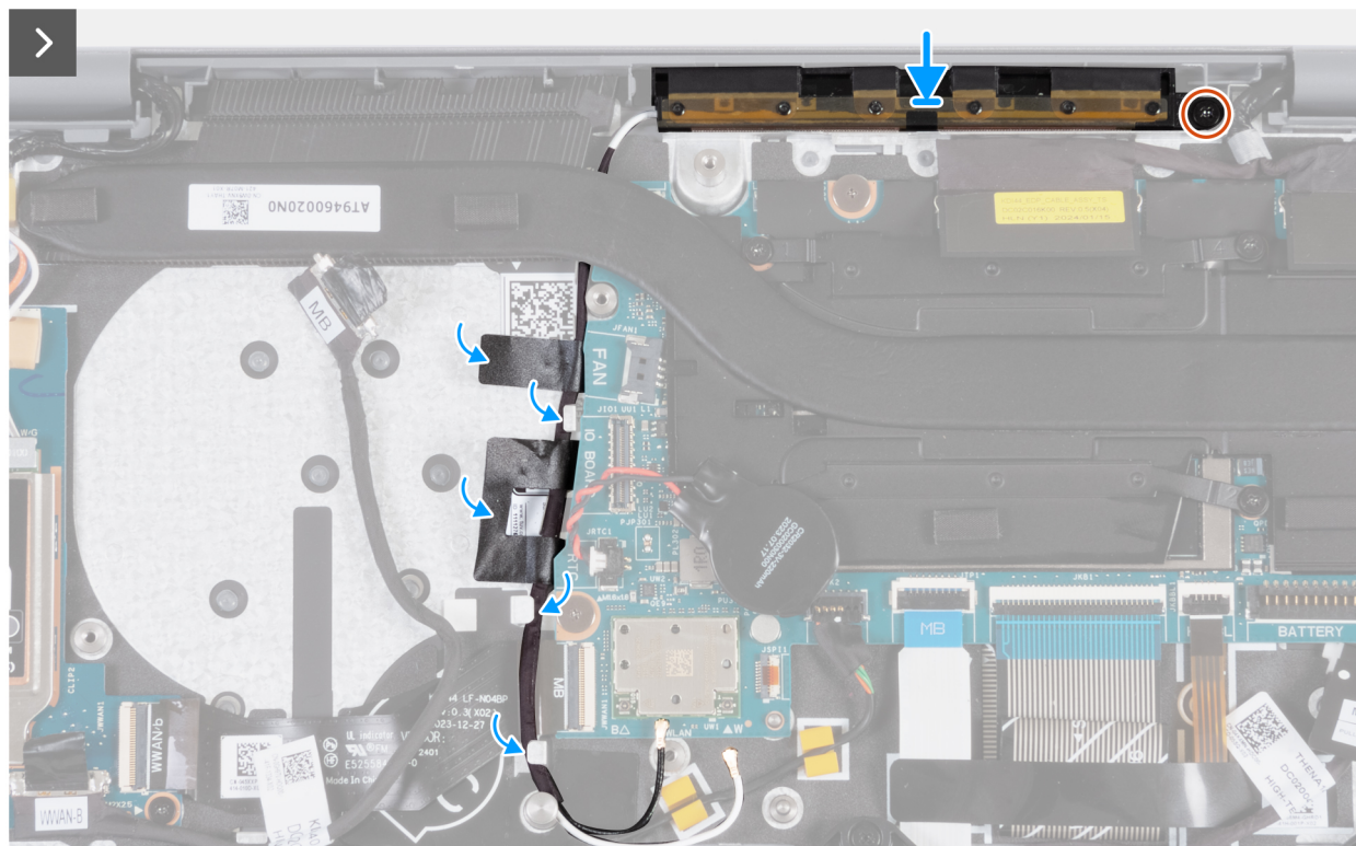
Abbildung 70. Installieren des WLAN-Antennenmoduls (bei Computern mit WWAN-Unterstützung)
