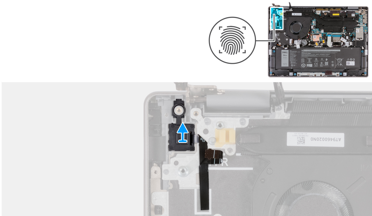
Abbildung 90. Entfernen des Netzschalters mit Fingerabdruck-Lesegerät
