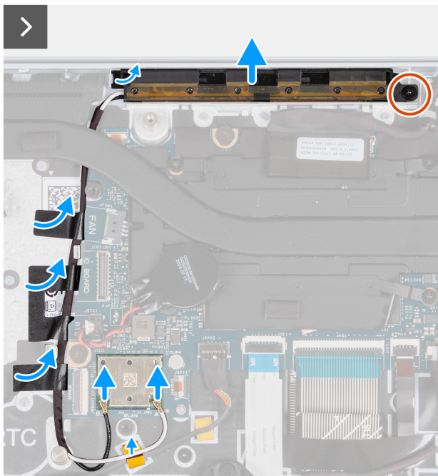
Abbildung 59. Entfernen des WLAN-Antennenmoduls (bei Computern nur mit WLAN-Unterstützung)
