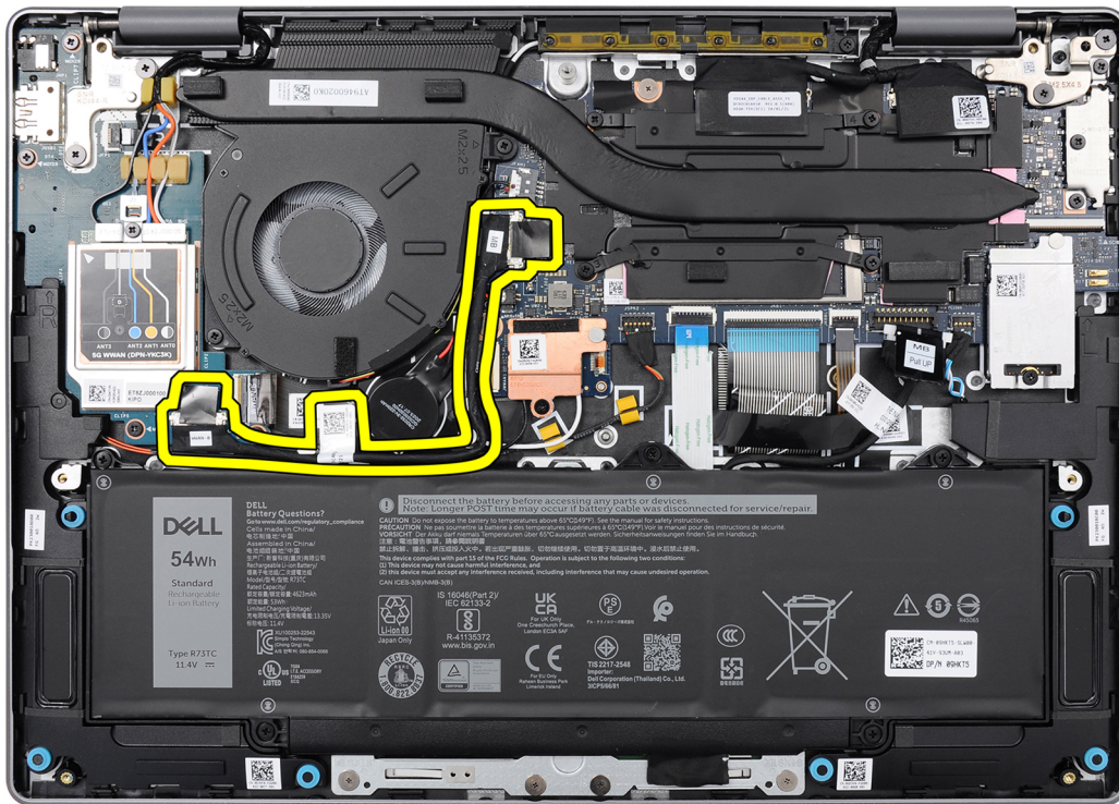
Abbildung 53. Position des I/O-Platinenkabels
