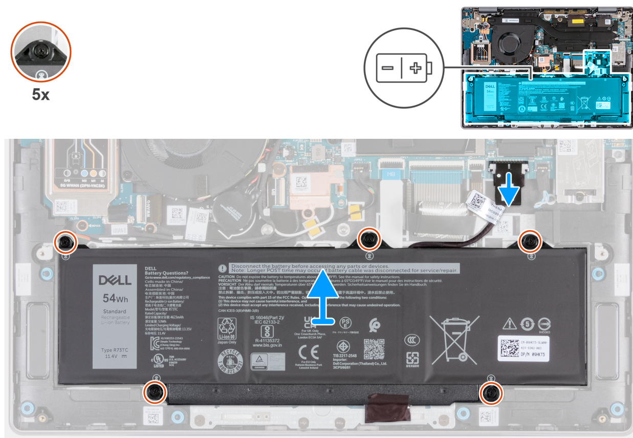
Abbildung 40. Entfernen des Akkus
