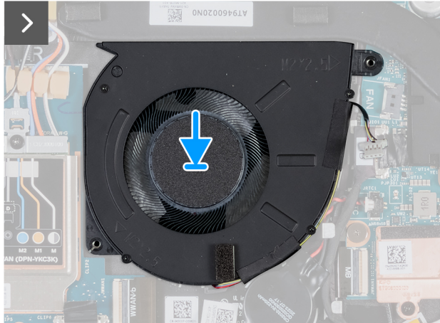
Abbildung 39. Installieren des Lüfters (Computer mit WWAN-Unterstützung)
