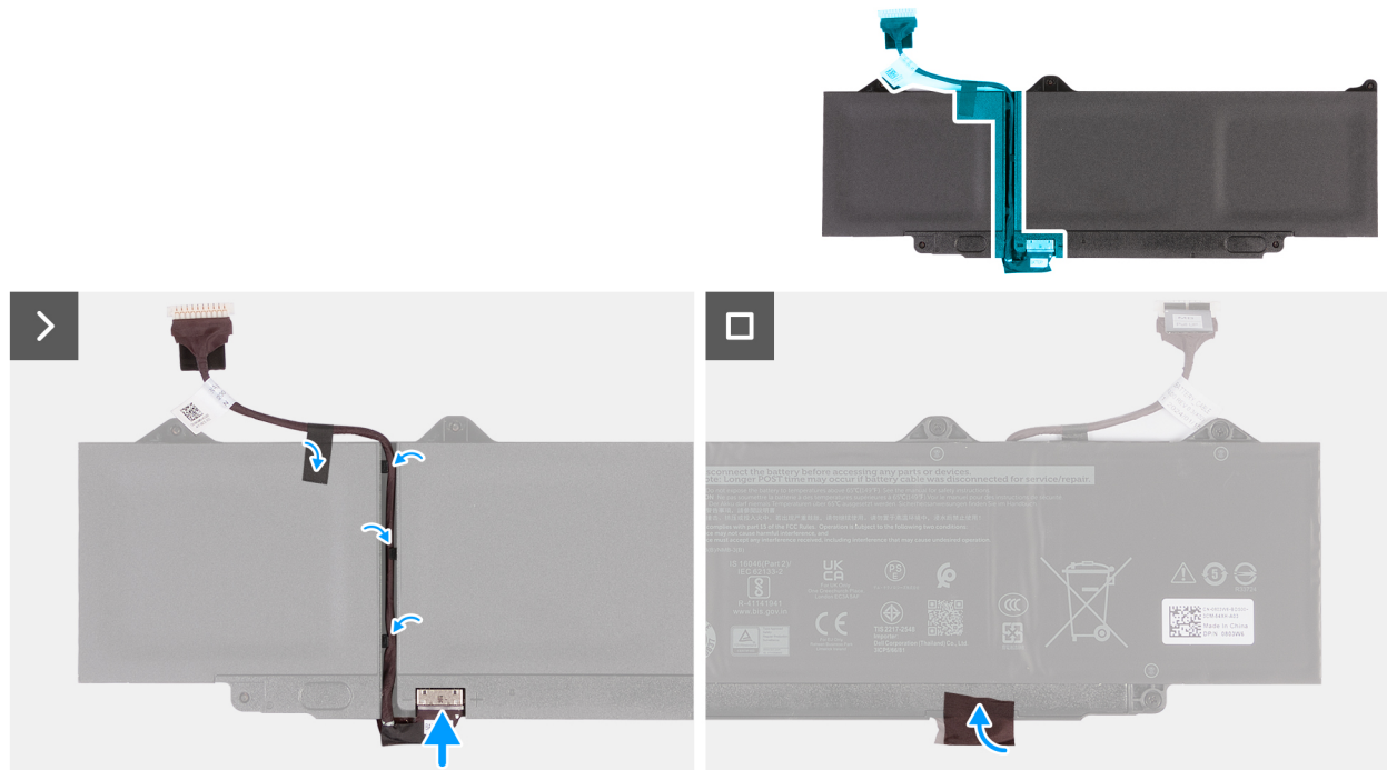
Abbildung 44. Einsetzen des Akkukabels
