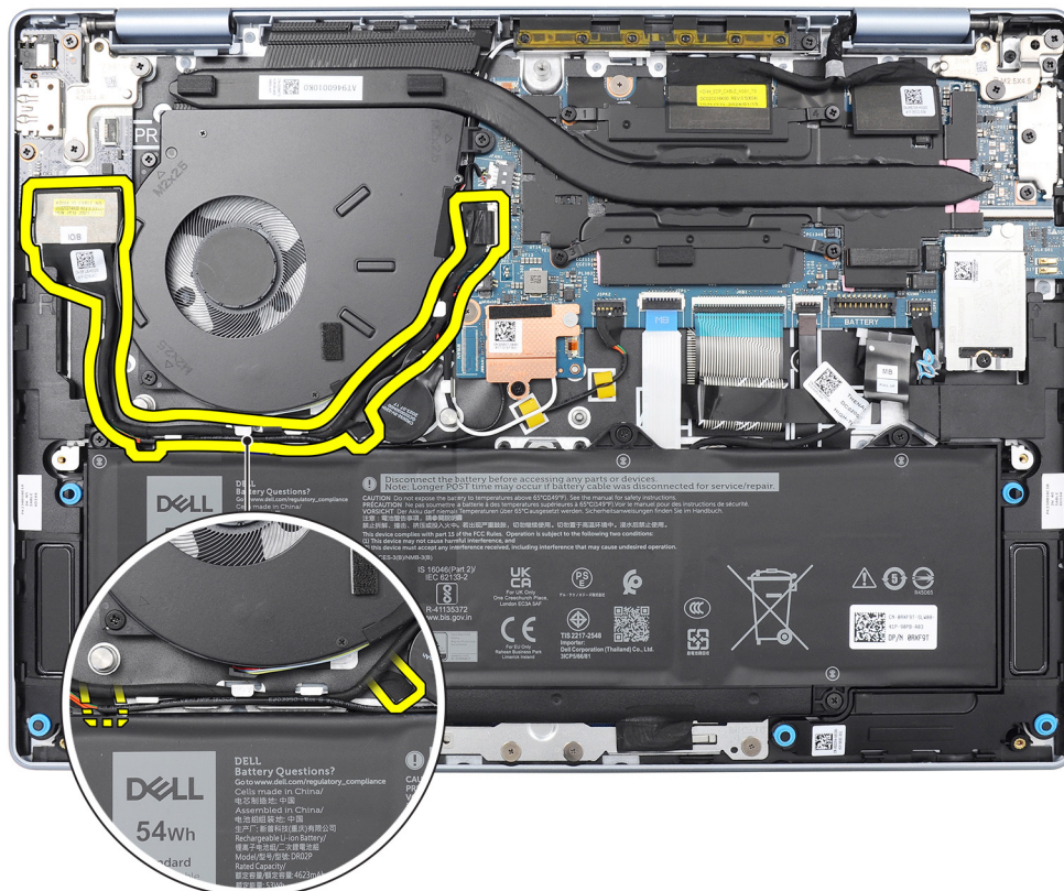
Abbildung 51. Position des I/O-Platinenkabels
