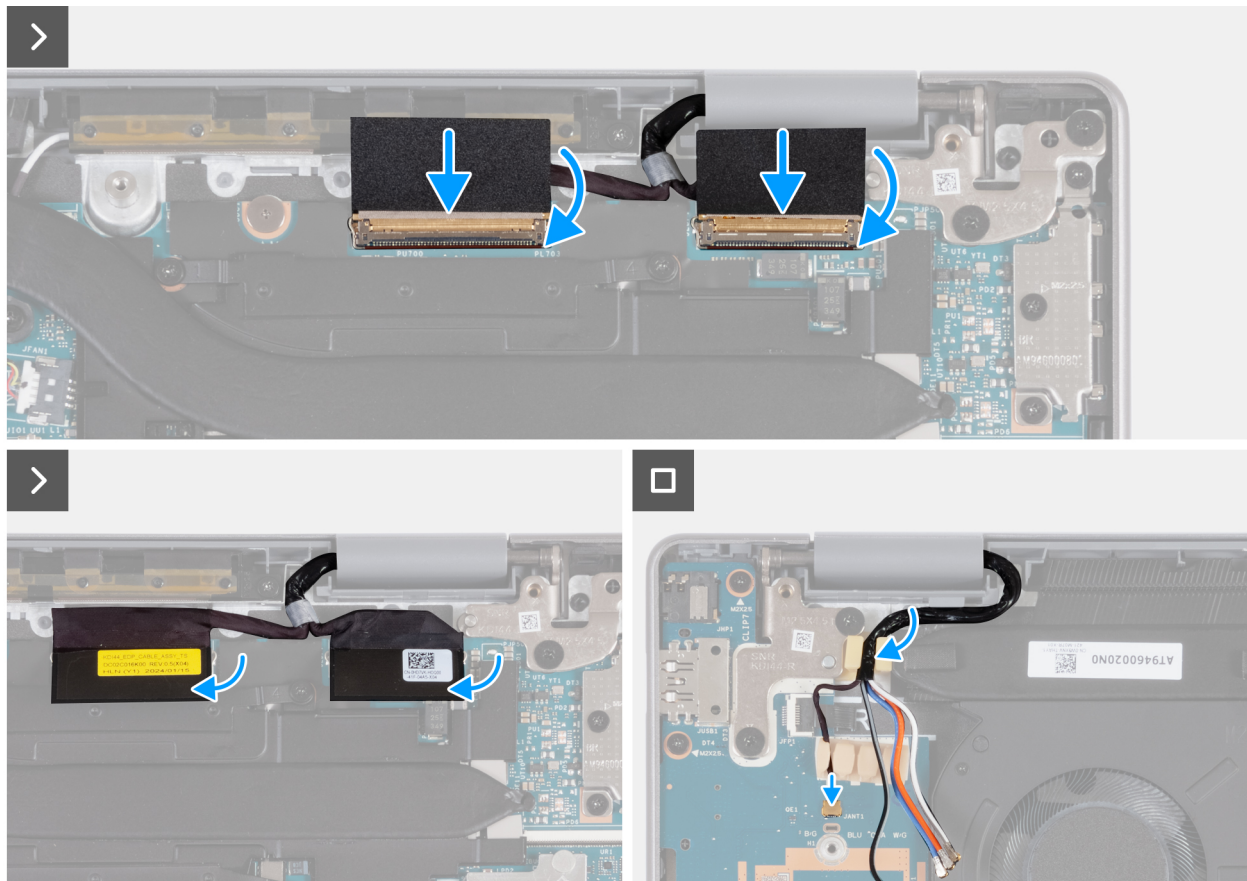
Abbildung 82. Einbauen der Bildschirmbaugruppe (bei Computern mit WWAN-Unterstützung)
