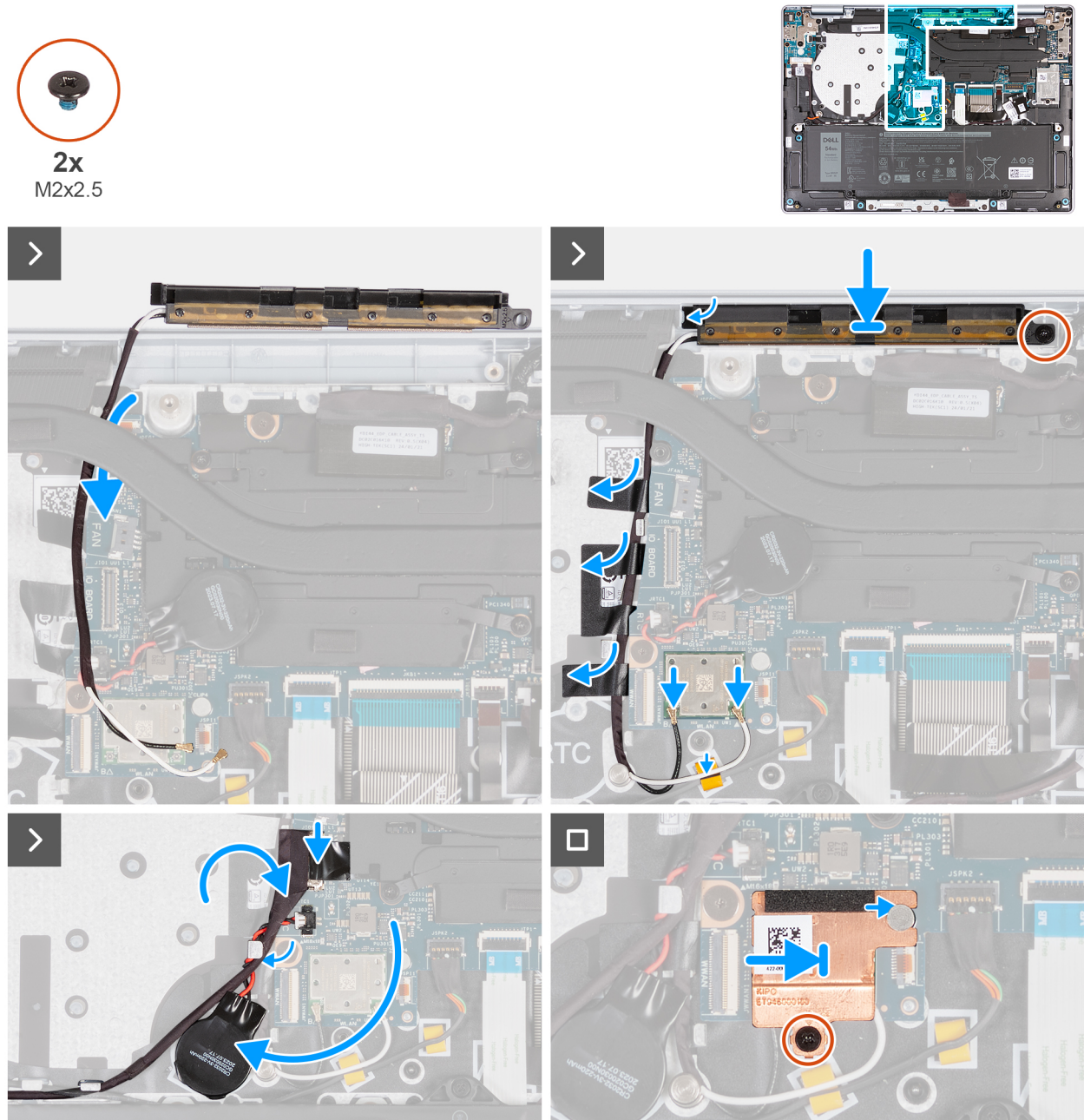
Abbildung 62. Installieren des WLAN-Antennenmoduls (bei Computern nur mit WLAN-Unterstützung)
