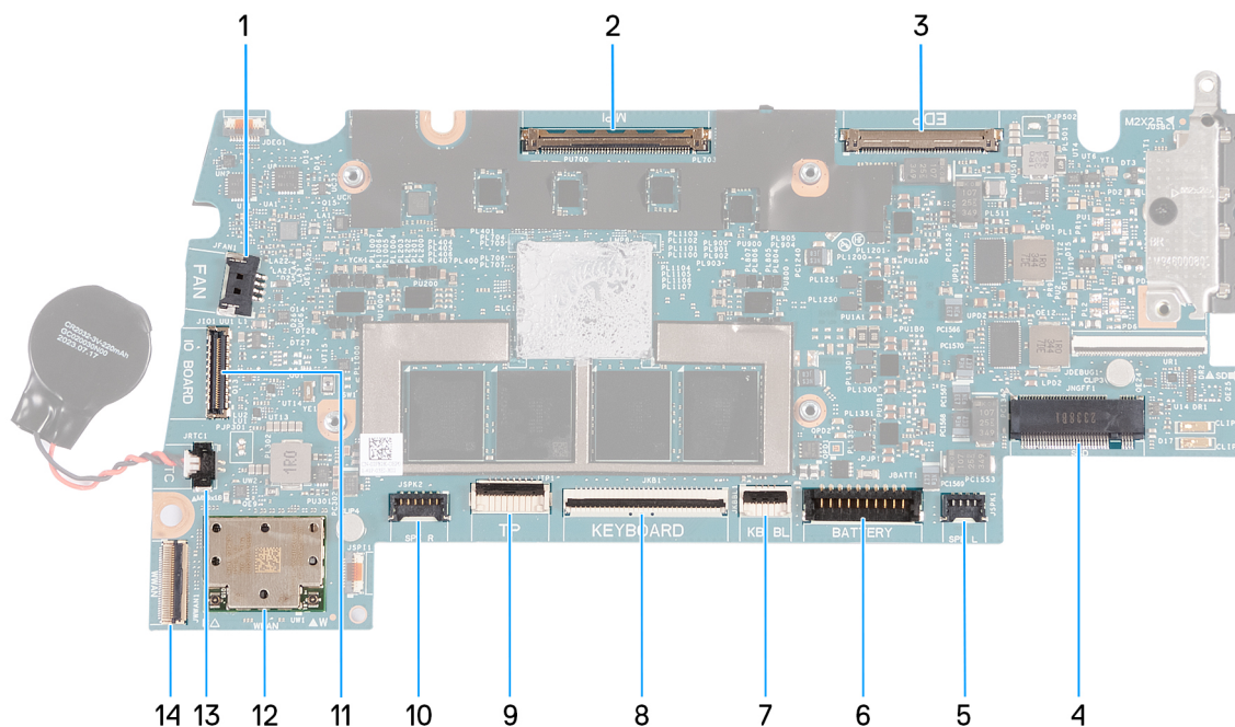
Abbildung 94. Hauptplattenanschlüsse
