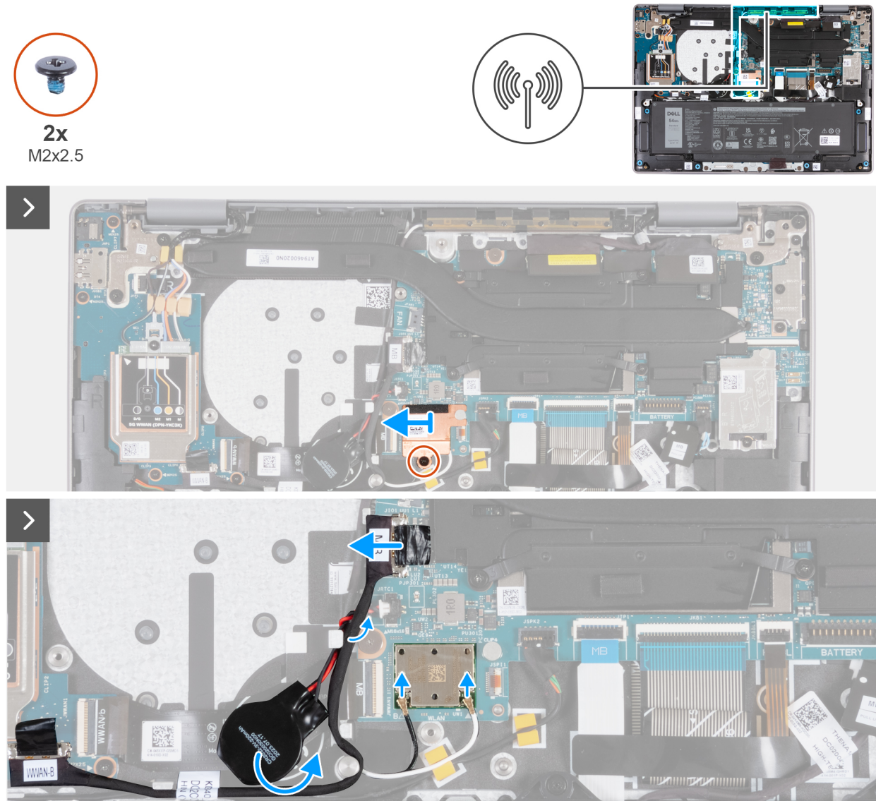
Abbildung 66. Entfernen des WLAN-Antennenmoduls
