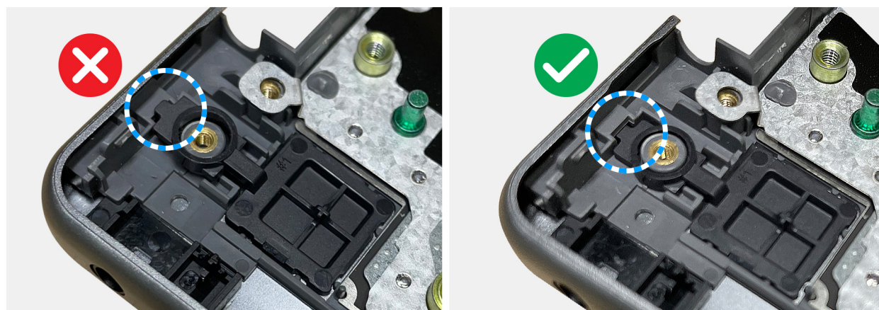
Abbildung 93. Einbauen des Netzschalters
