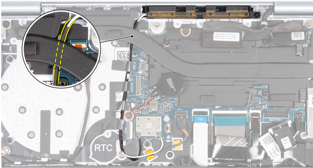
Abbildung 69. Entfernen der WLAN-Antennenkabel
