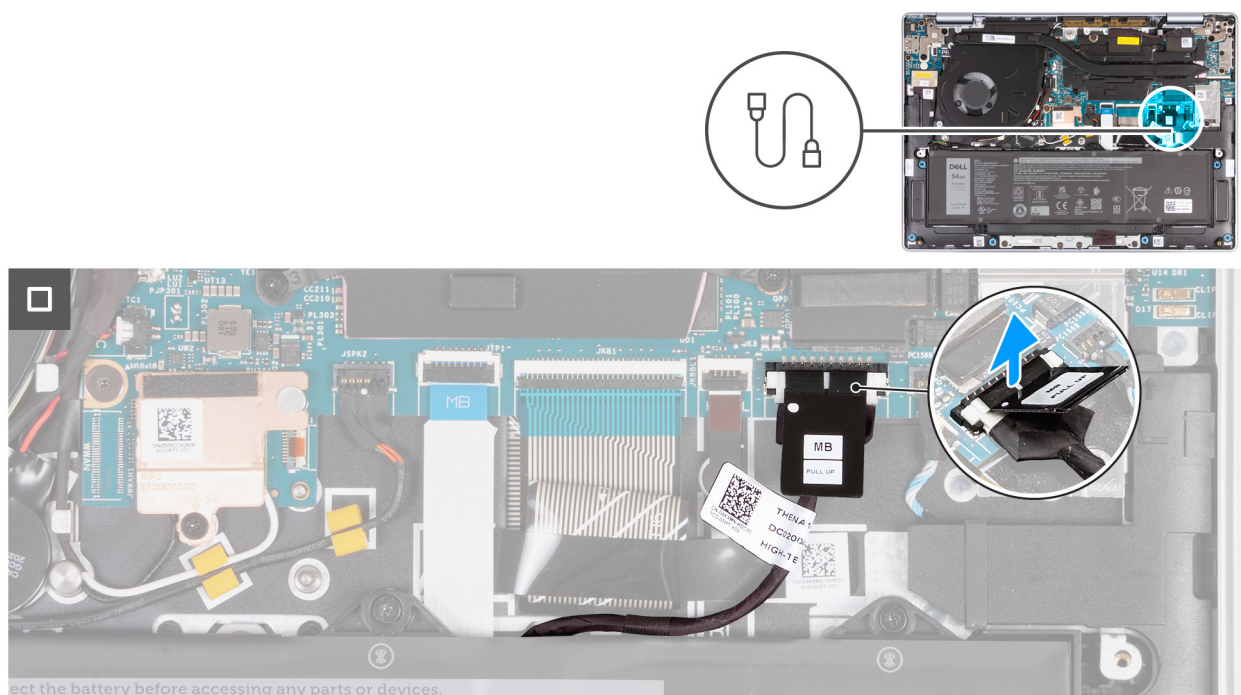
Abbildung 18. Trennen des Batteriekabels.
