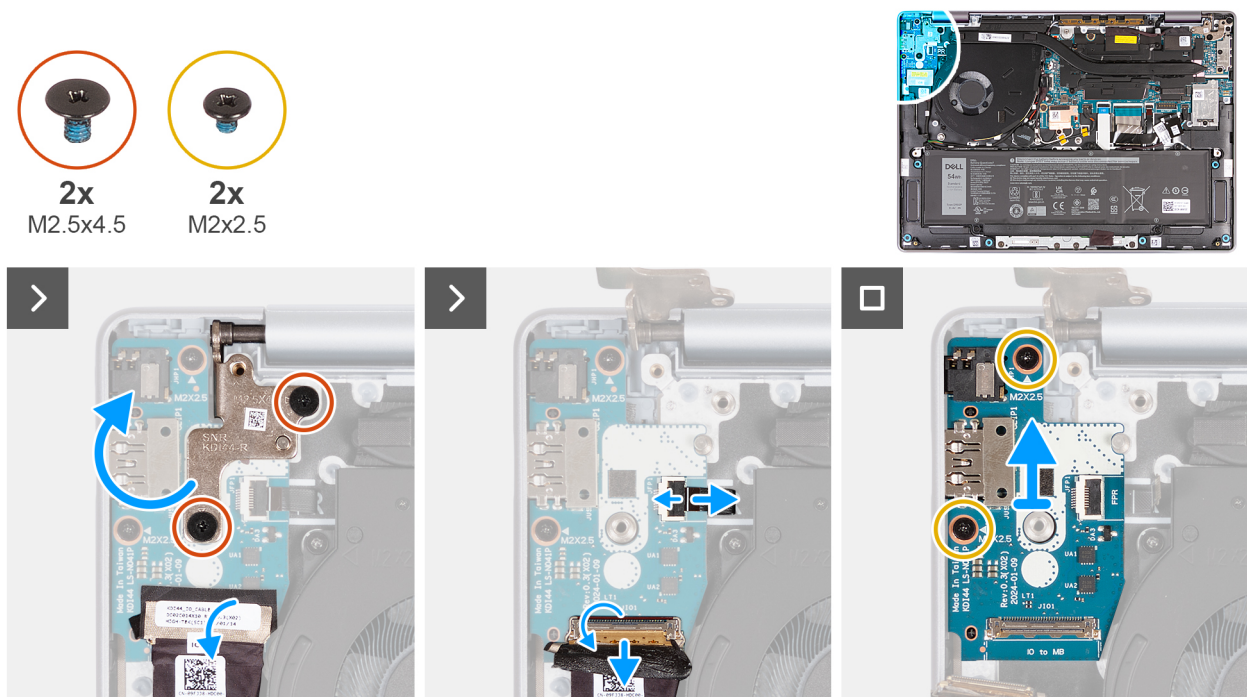
Abbildung 83. Entfernen der I/O-Platine (bei Computern nur mit WLAN-Unterstützung)
