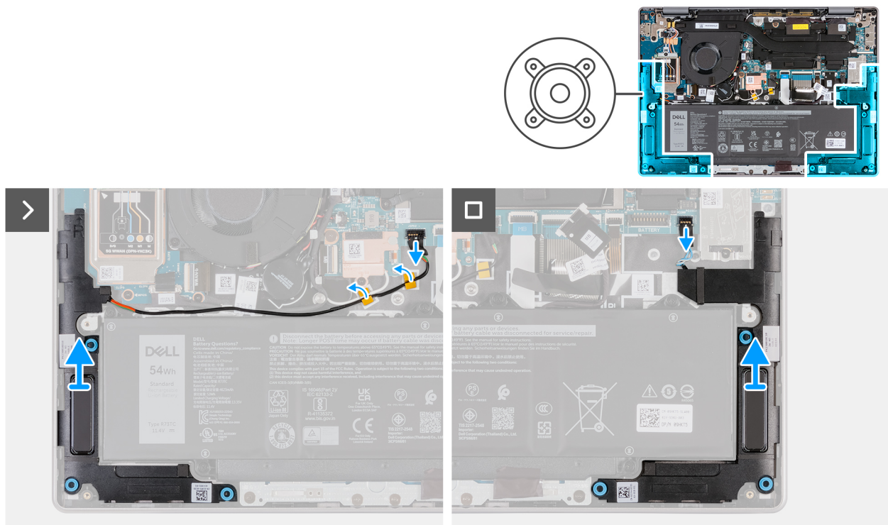
Abbildung 32. Entfernung der Lautsprecher
