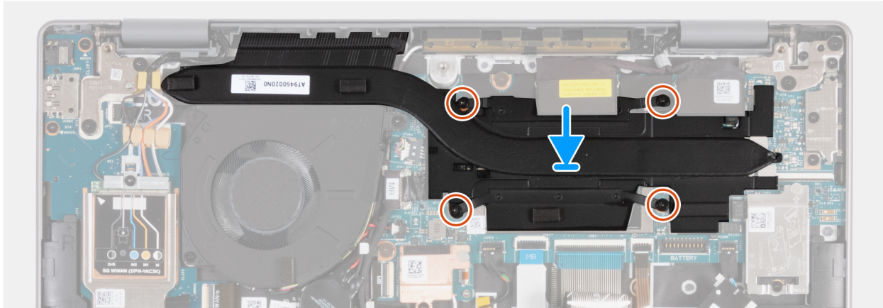
Abbildung 46. Einsetzen des Kühlkörpers
