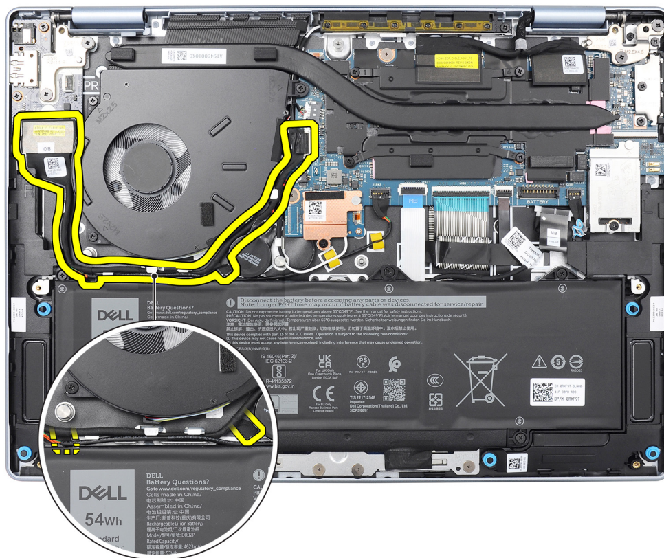
Abbildung 49. Position des I/O-Platinenkabels
