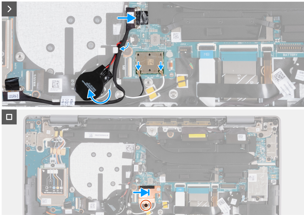
Abbildung 71. Installieren des WLAN-Antennenmoduls (bei Computern mit WWAN-Unterstützung)
