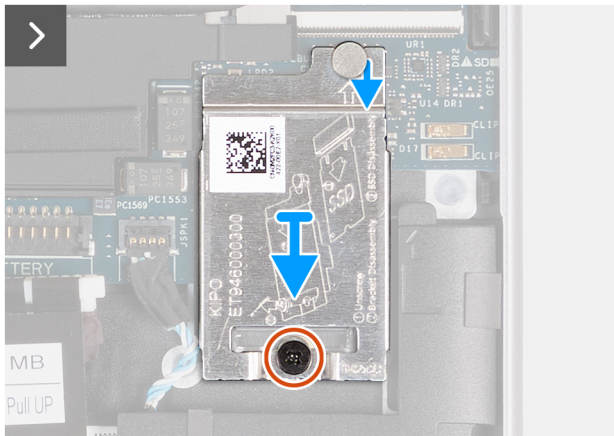
Abbildung 22. Entfernen der SSD
