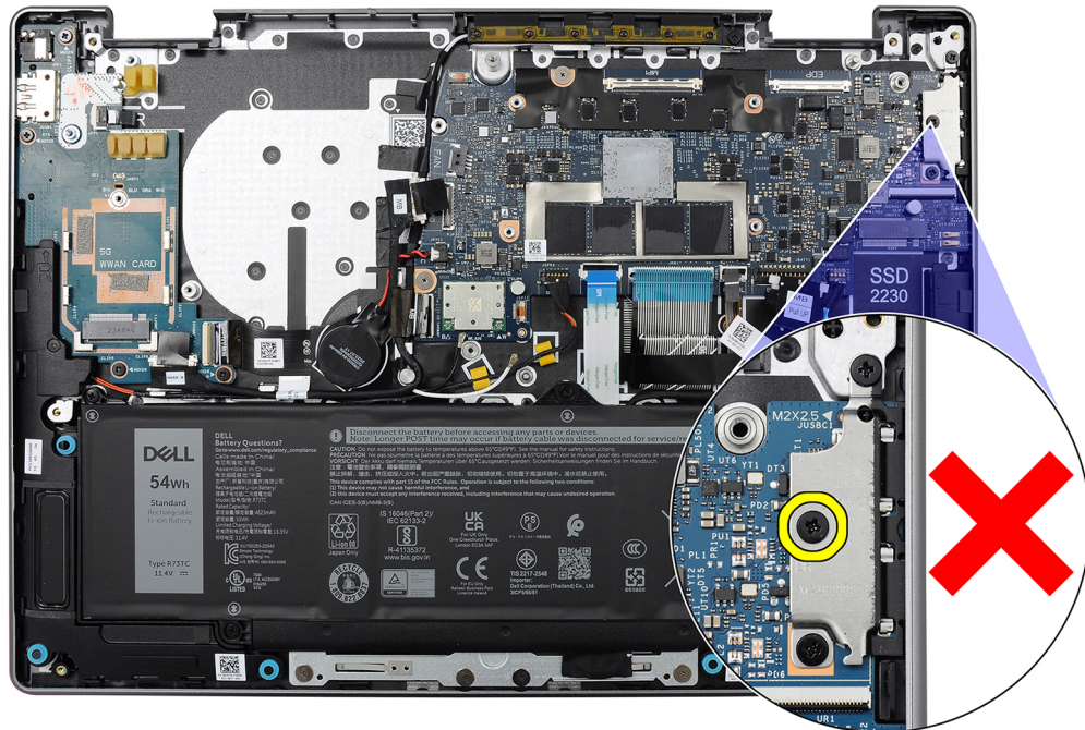
Abbildung 97. USB-Typ-C-Halterung
