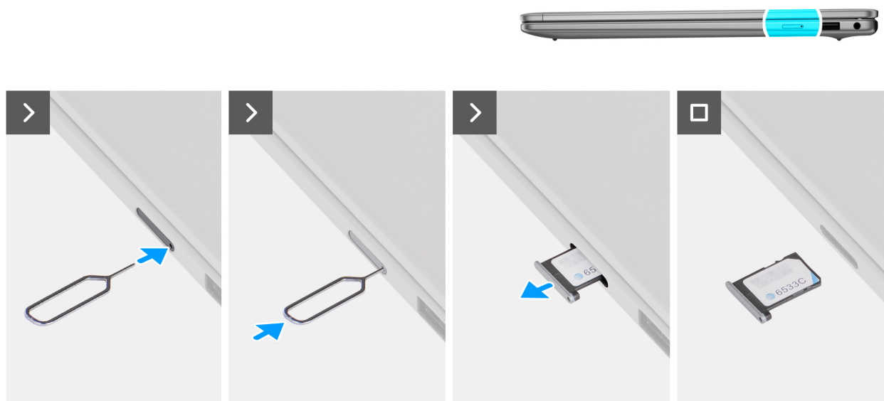
Abbildung 14. Entfernen des SIM-Kartenfachs
