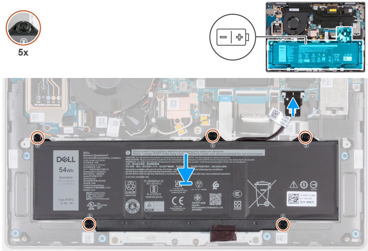
Abbildung 41. Einsetzen des Akkus
