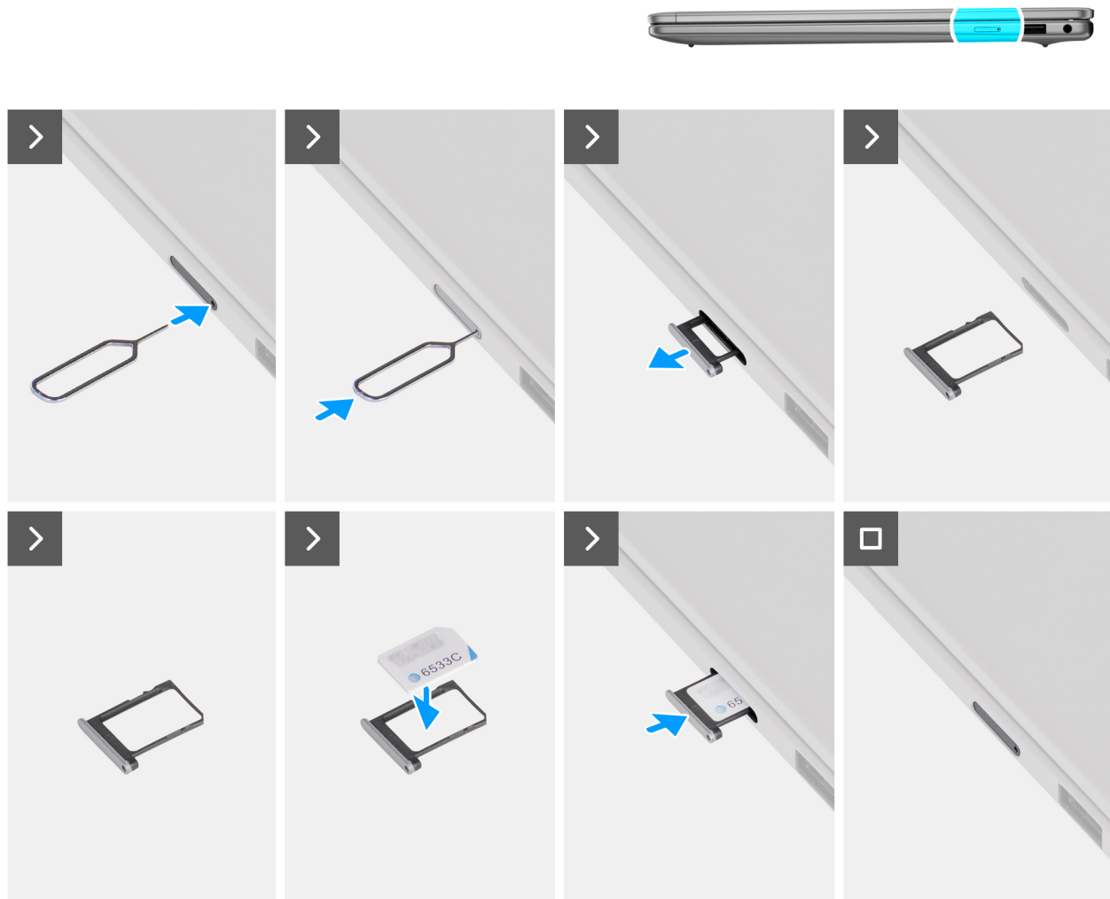
Abbildung 13. Installieren der SIM-Karte
