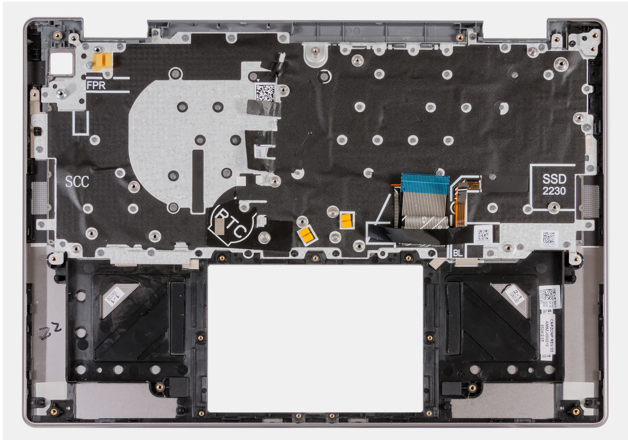
Abbildung 102. Handballenstützen- und Tastaturbaugruppe
