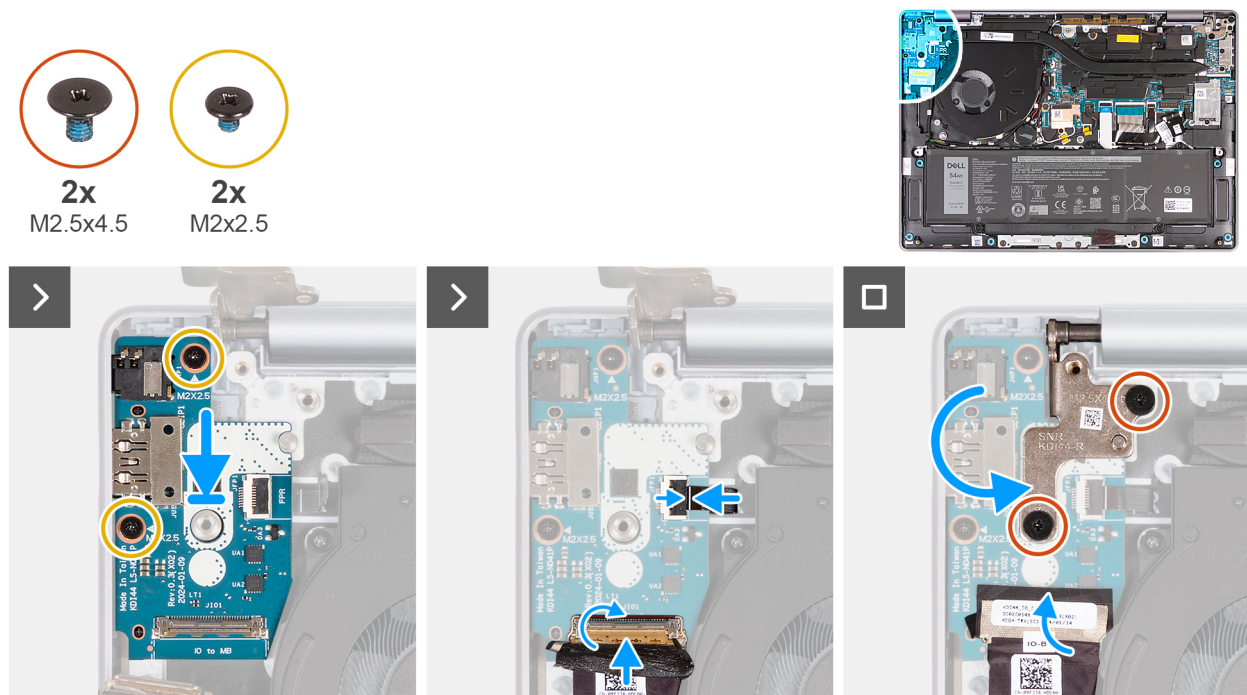
Abbildung 84. Installation der I/O-Platine (bei Computern nur mit WLAN-Unterstützung)
