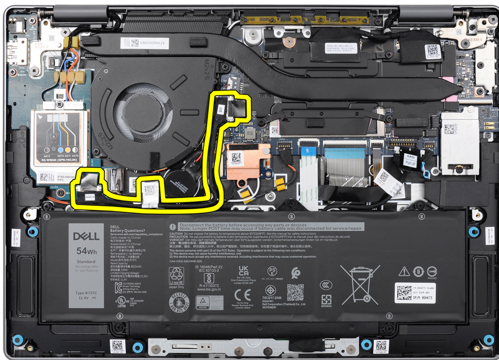
Abbildung 55. Position des I/O-Platinenkabels
