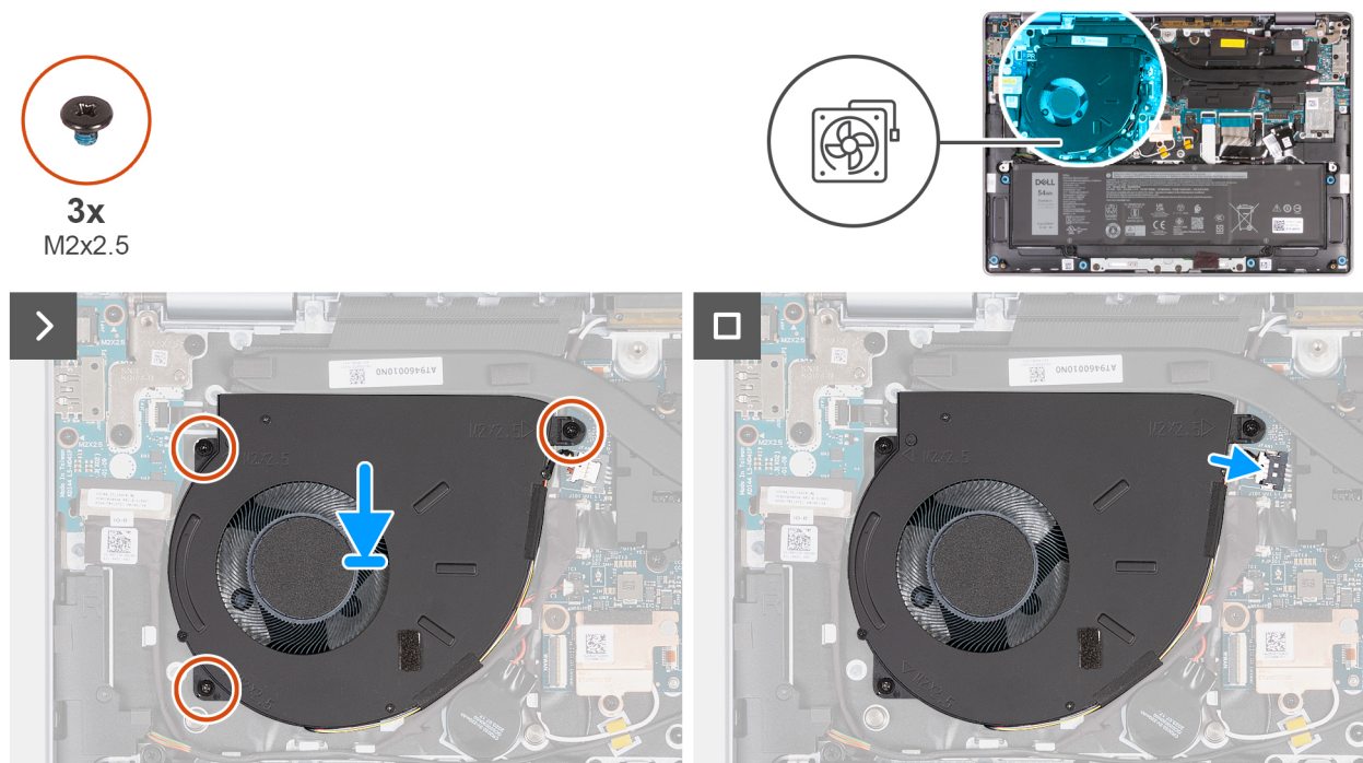
Abbildung 37. Installieren des Lüfters (bei Computern nur mit WLAN-Unterstützung)
