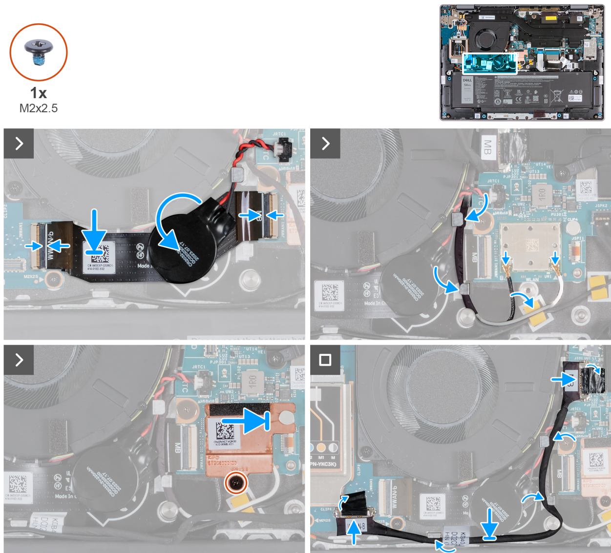
Abbildung 58. Installieren des FPC-Kabels der I/O-Platine
