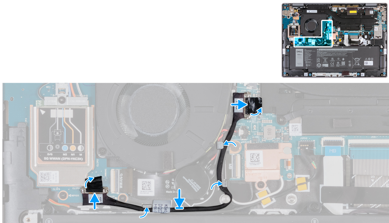
Abbildung 56. Installieren des I/O-Platinenkabels (Computer mit WWAN-Unterstützung)
