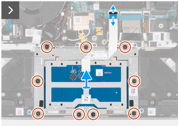
Abbildung 87. Entfernen der Touchpad-Baugruppe
