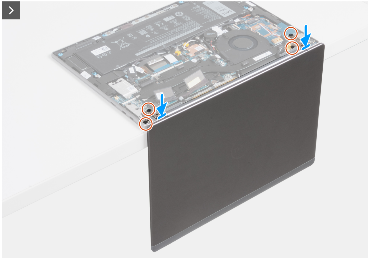
Abbildung 81. Einbauen der Bildschirmbaugruppe (bei Computern mit WWAN-Unterstützung)
