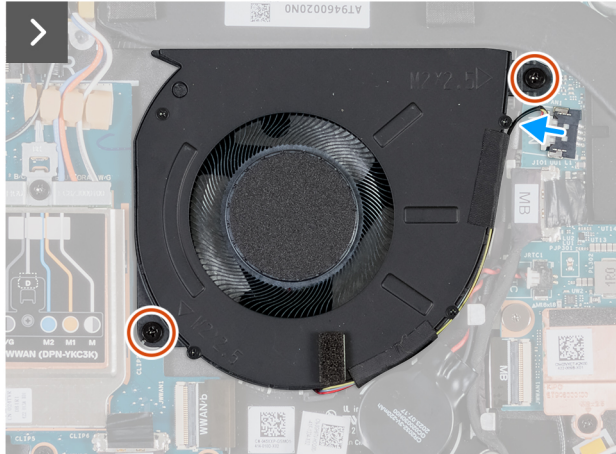
Abbildung 38. Entfernen des Lüfters (Computer mit WWAN-Unterstützung)
