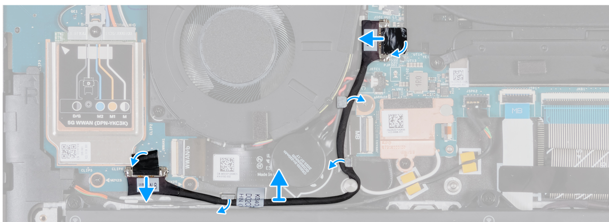
Abbildung 54. Entfernen des I/O-Platinenkabels (Computer mit WWAN-Unterstützung)
