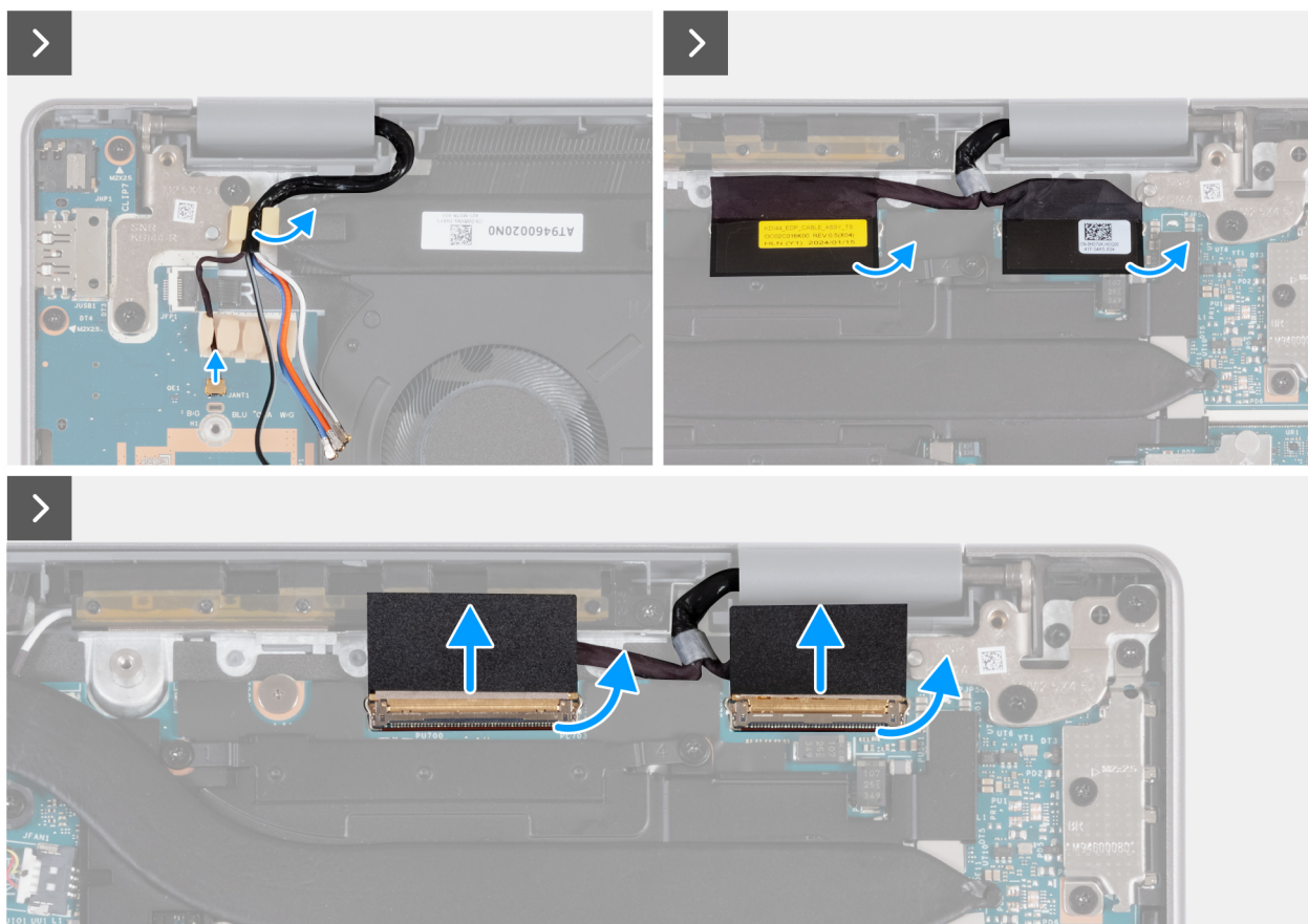
Abbildung 78. Entfernen der Bildschirmbaugruppe (bei Computern mit WWAN-Unterstützung)
