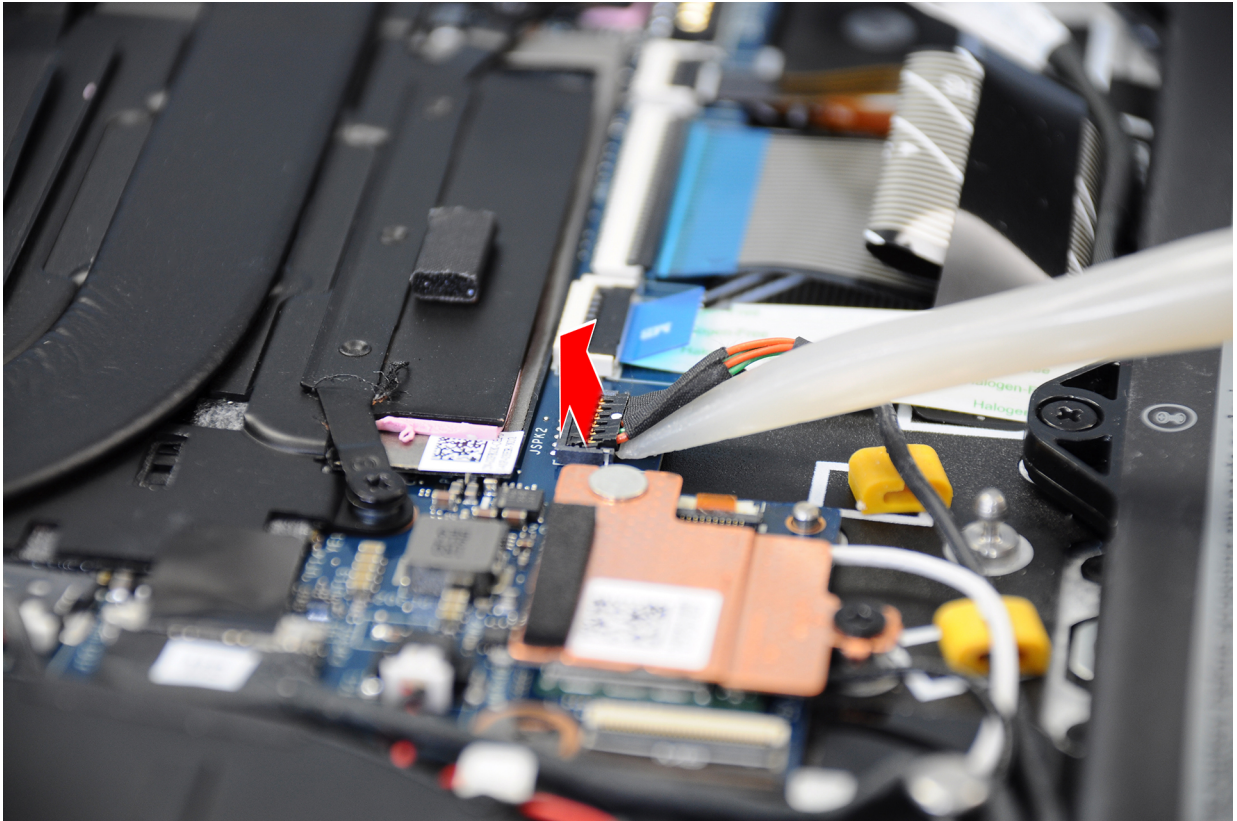
Abbildung 33. Hebeln Sie das Lautsprecherkabel vom Anschluss ab
