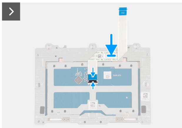
Abbildung 88. Installieren der Touchpad-Baugruppe
