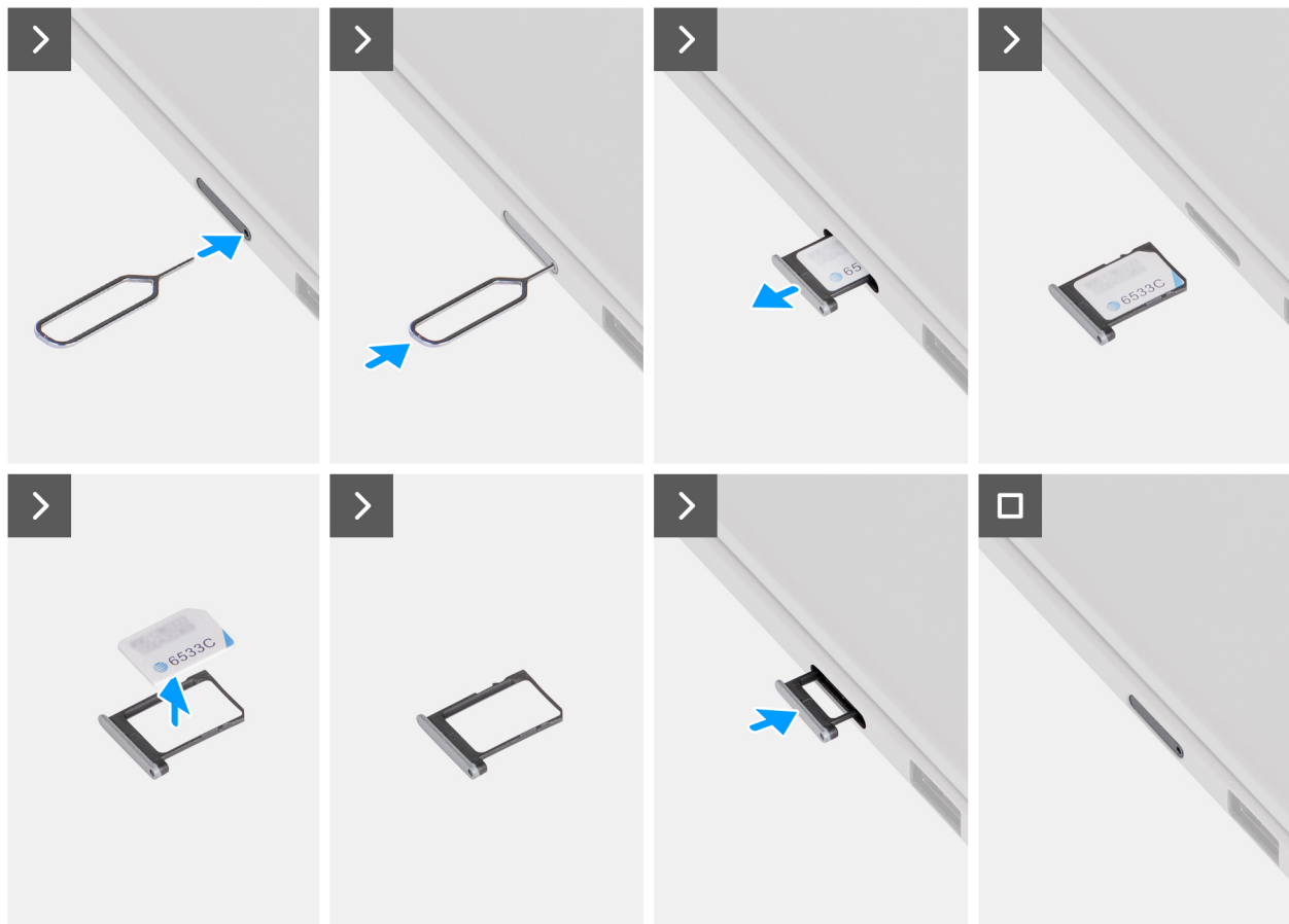
Abbildung 12. Entfernen der SIM-Karte
