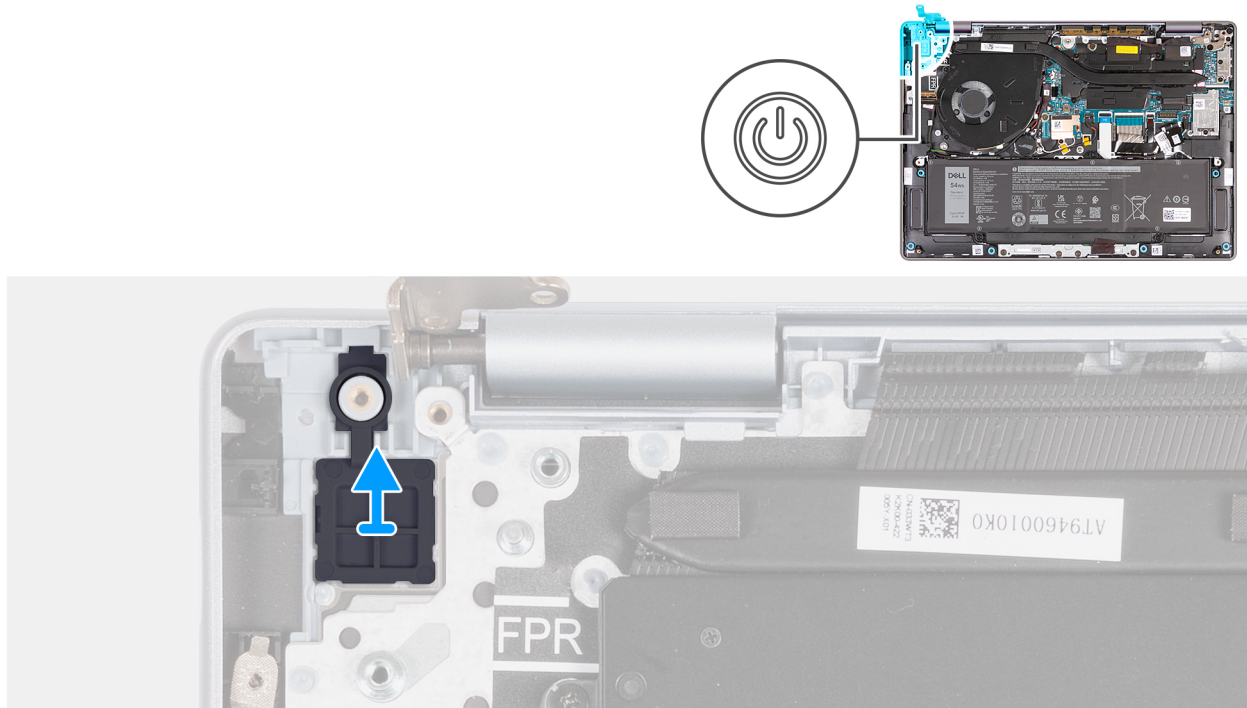
Abbildung 89. Entfernen des Netzschalters
