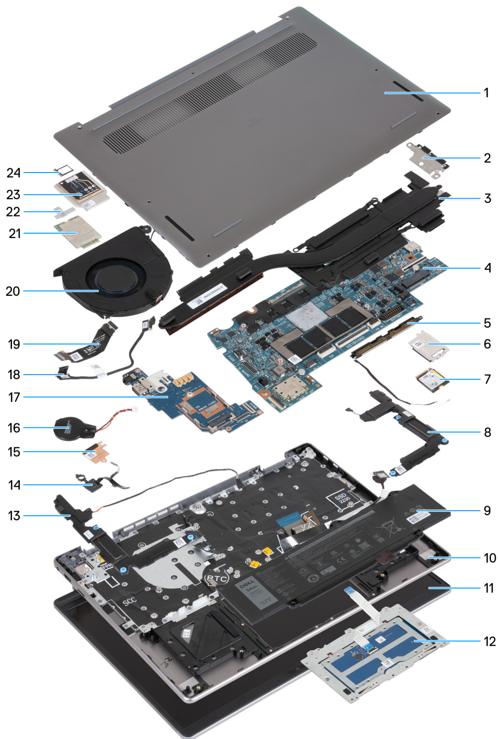
Abbildung 11. Hauptkomponenten des Latitude 7455 (Computer mit WWAN-Unterstützung)
