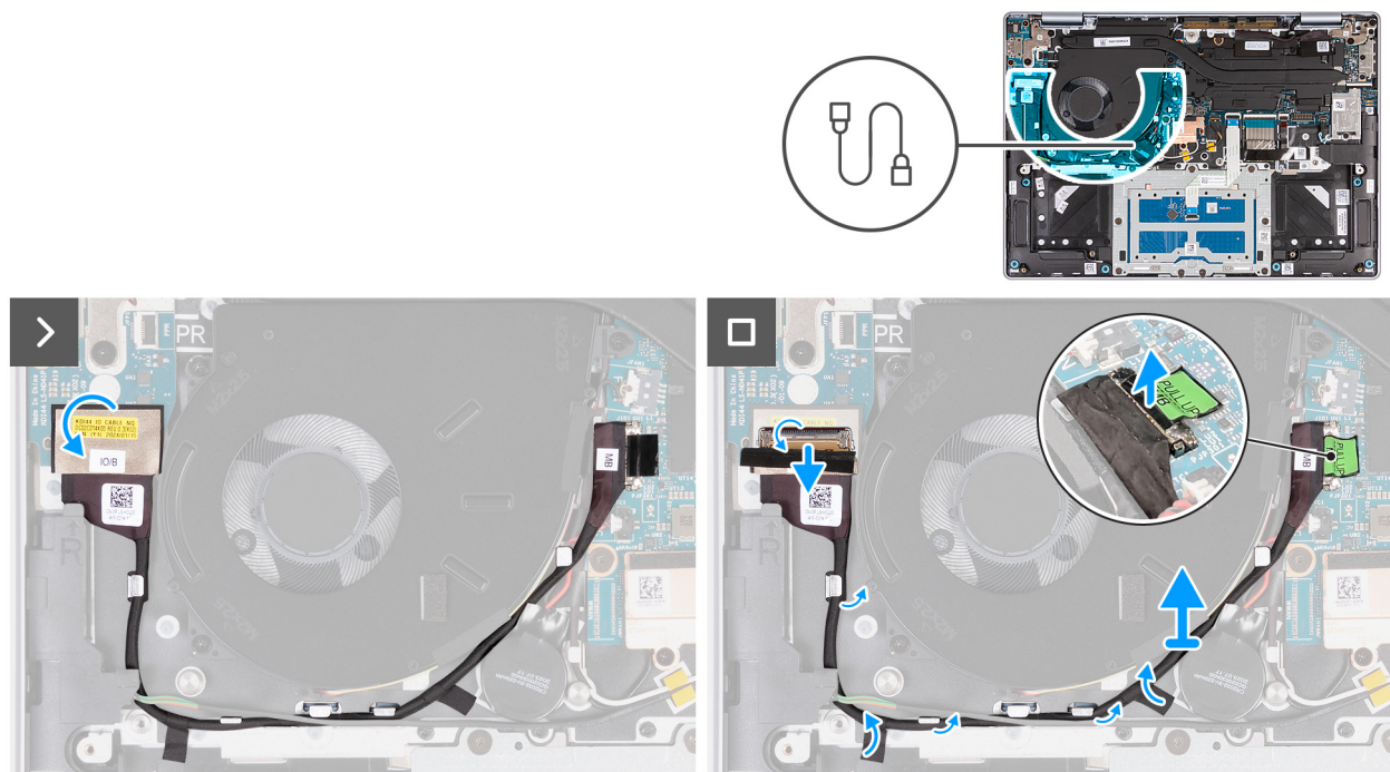
Abbildung 50. Entfernen des I/O-Platinenkabels (bei Computern mit WLAN-Unterstützung)
