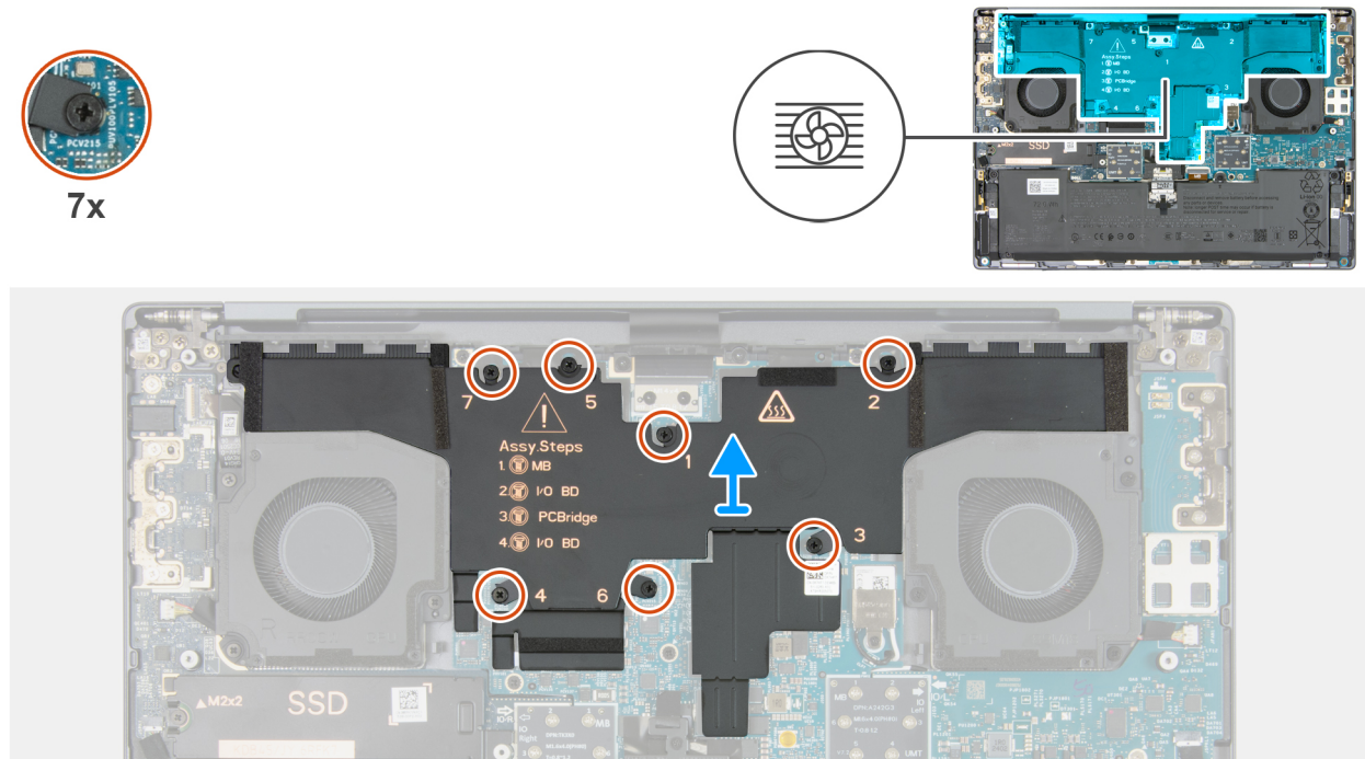
Abbildung 43. Kühlkörper entfernen
