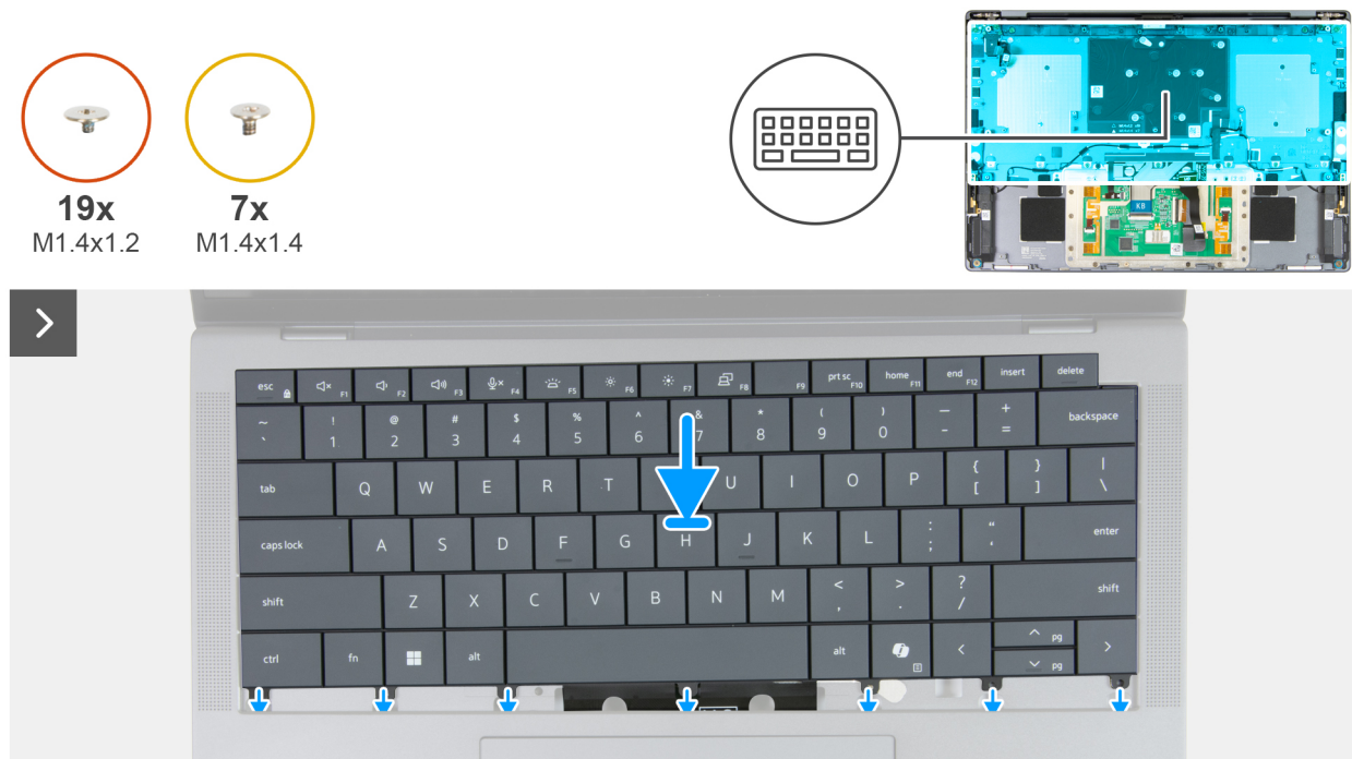
Abbildung 74. Einbauen der Tastatur
