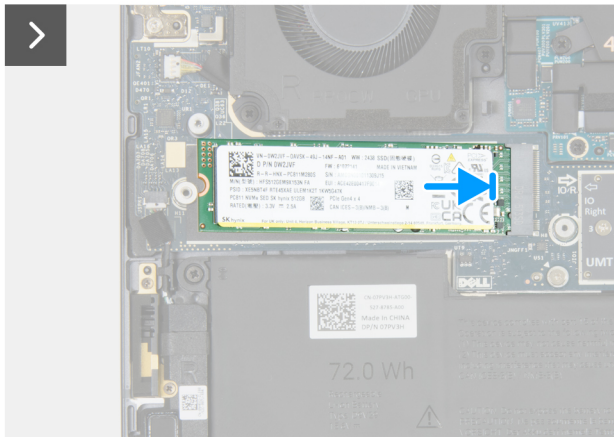
Abbildung 24. Installieren des M.2 2280-Solid-State-Laufwerks
