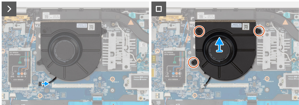
Abbildung 28. Entfernen des Lüfters
