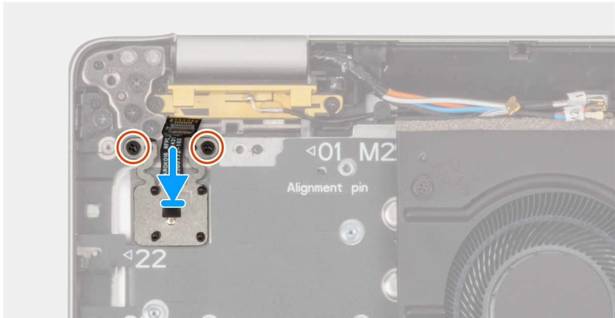
Abbildung 54. Installieren des Netzschalters mit optionalem Fingerabdruck-Lesegerät
