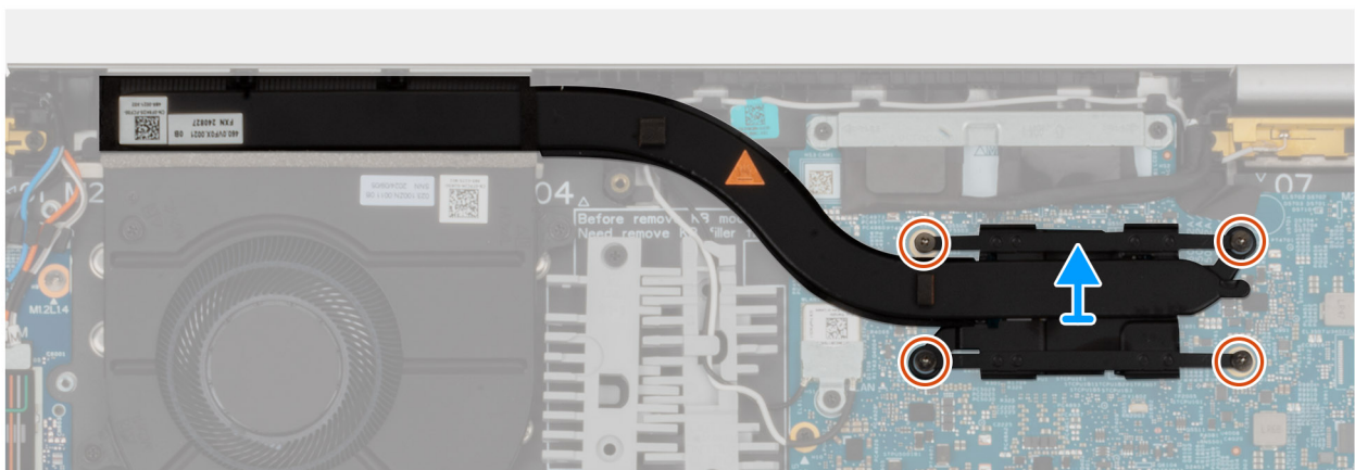
Abbildung 45. Kühlkörper entfernen
