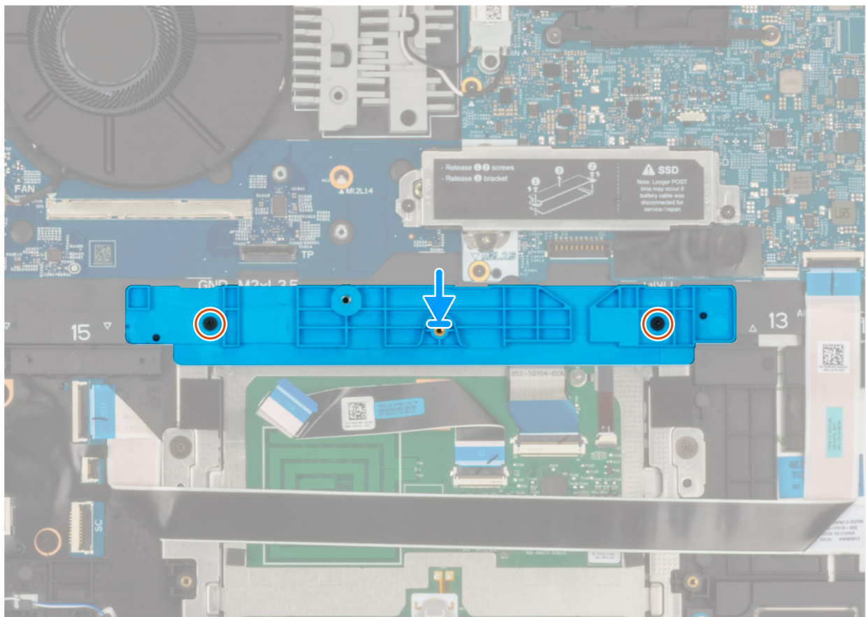
Abbildung 40. Installieren der Akkuhalterung
