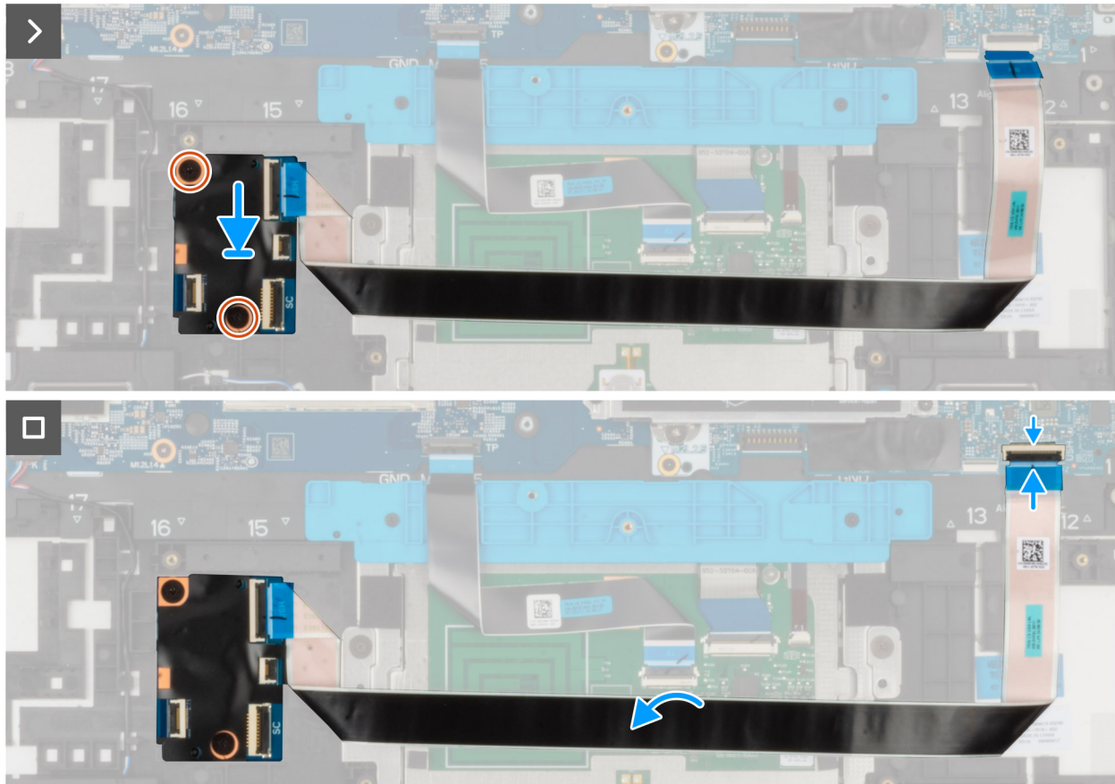
Abbildung 42. USH-Platine
