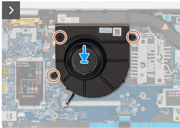
Abbildung 29. Einbauen des Lüfters
