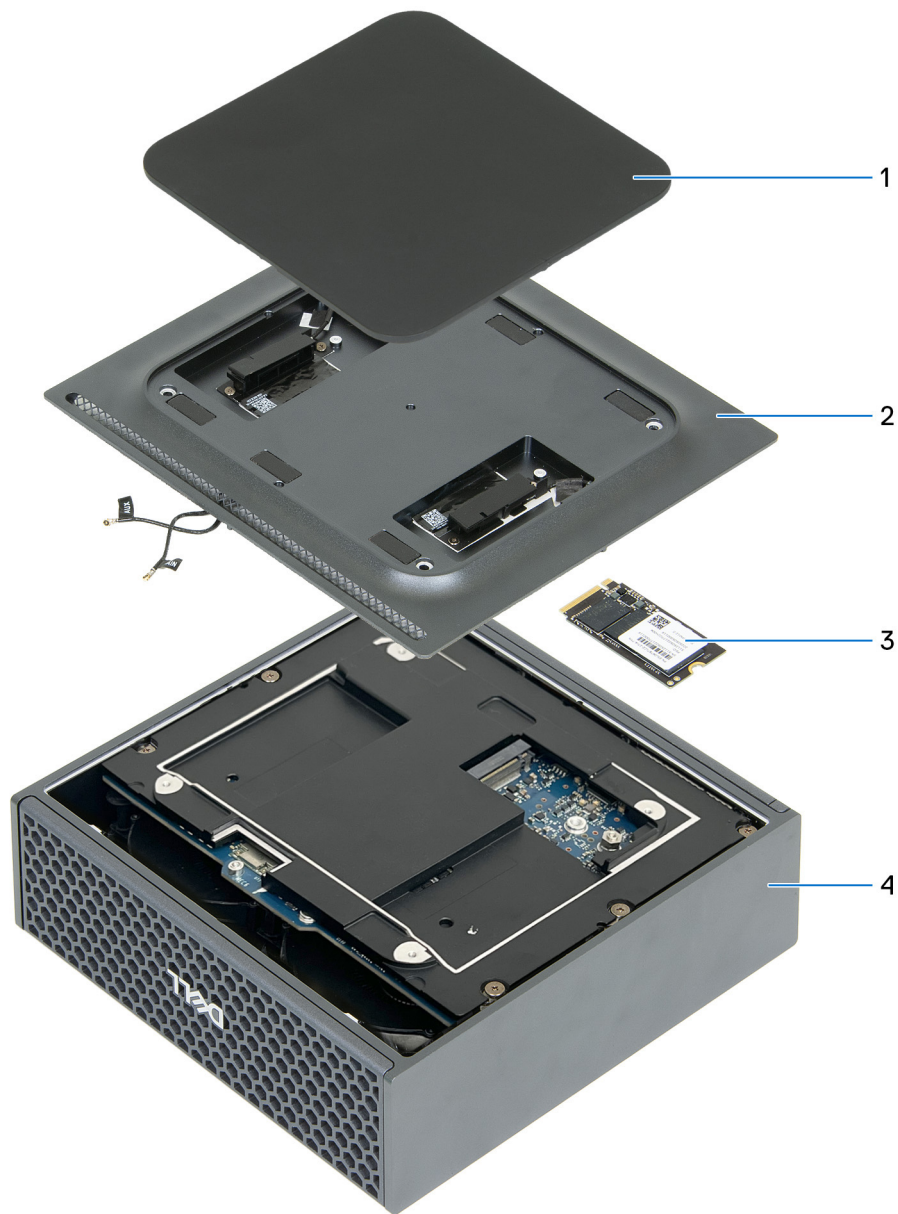
Abbildung 15. Hauptkomponenten von Dell Pro Max mit GB10
