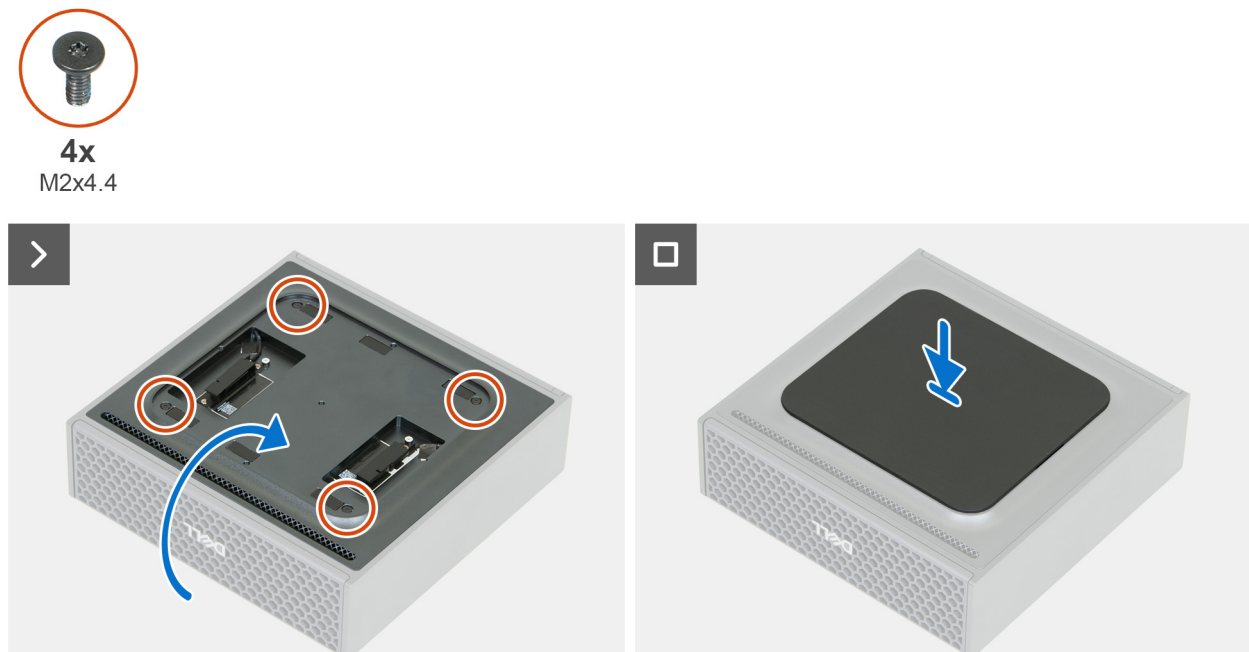
Abbildung 21. Vorbereiten des Computers auf die Rücksendung
