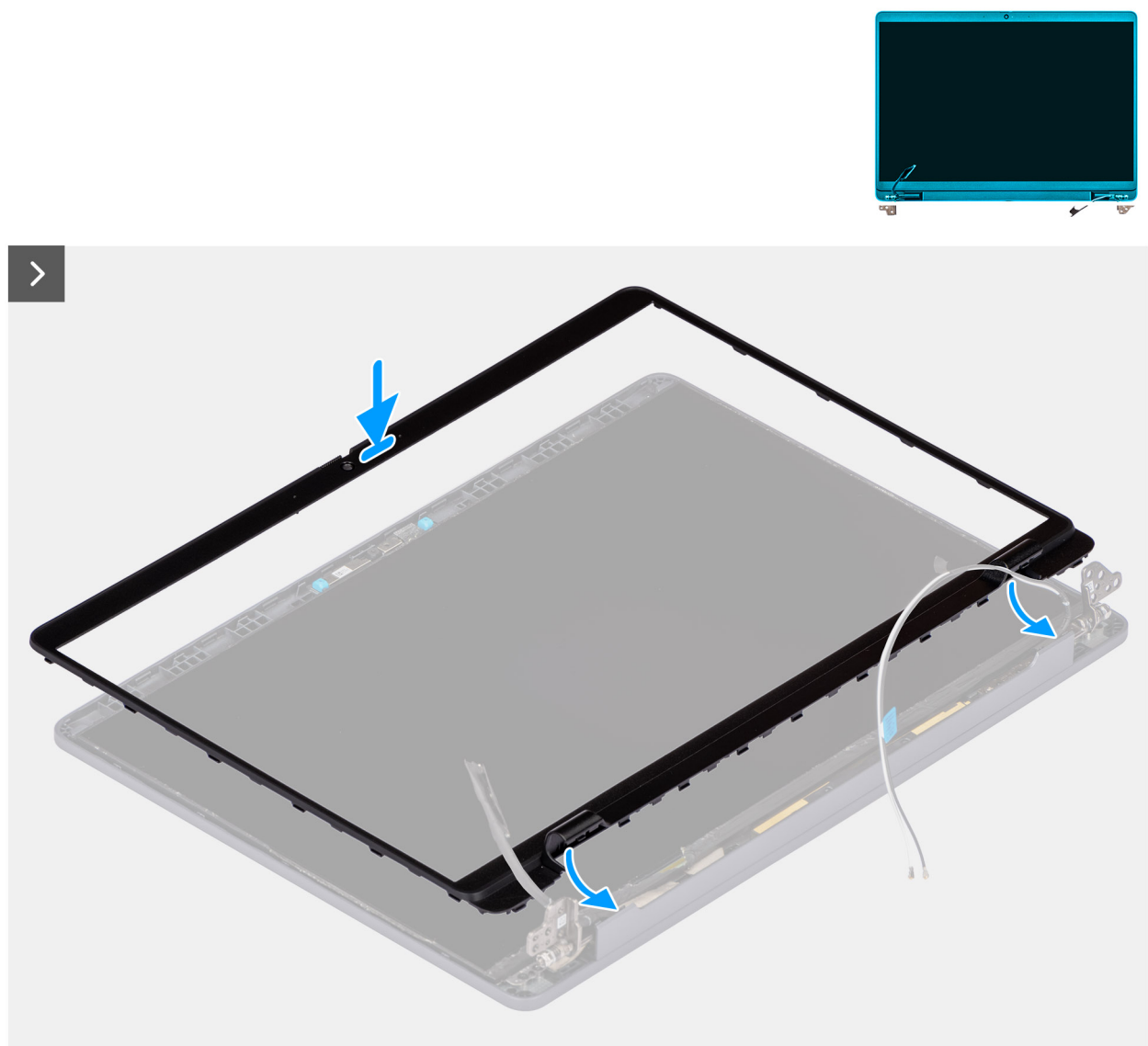
Abbildung 58. Installing the display bezel
