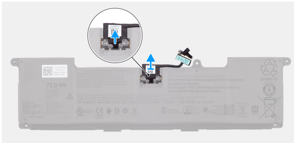
Abbildung 18. Trennen des Batteriekabels.
