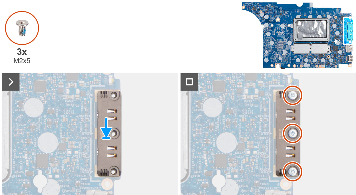
Abbildung 93. Installing the USB Type-C module
