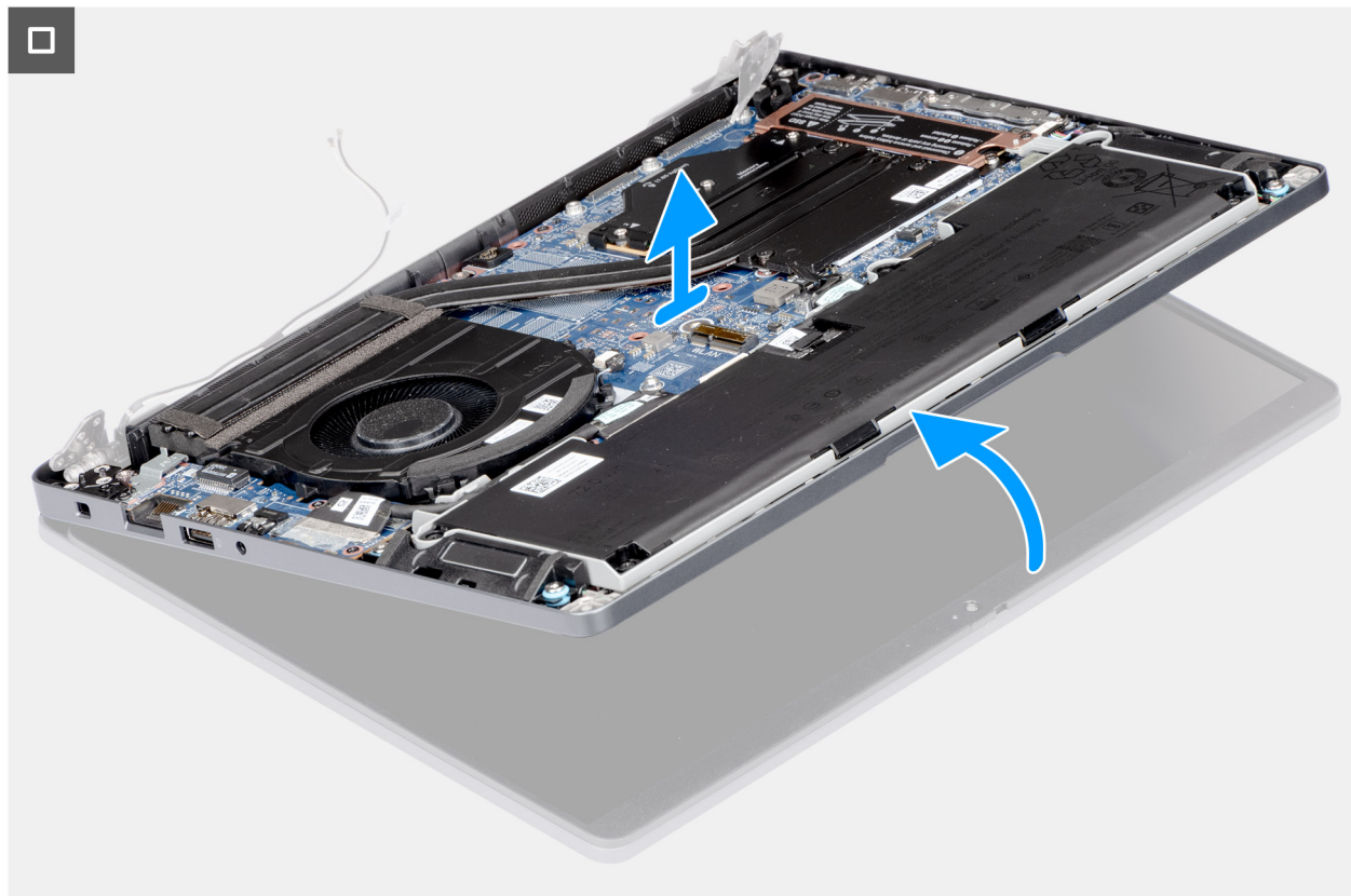
Abbildung 48. Entfernen der Bildschirmbaugruppe
