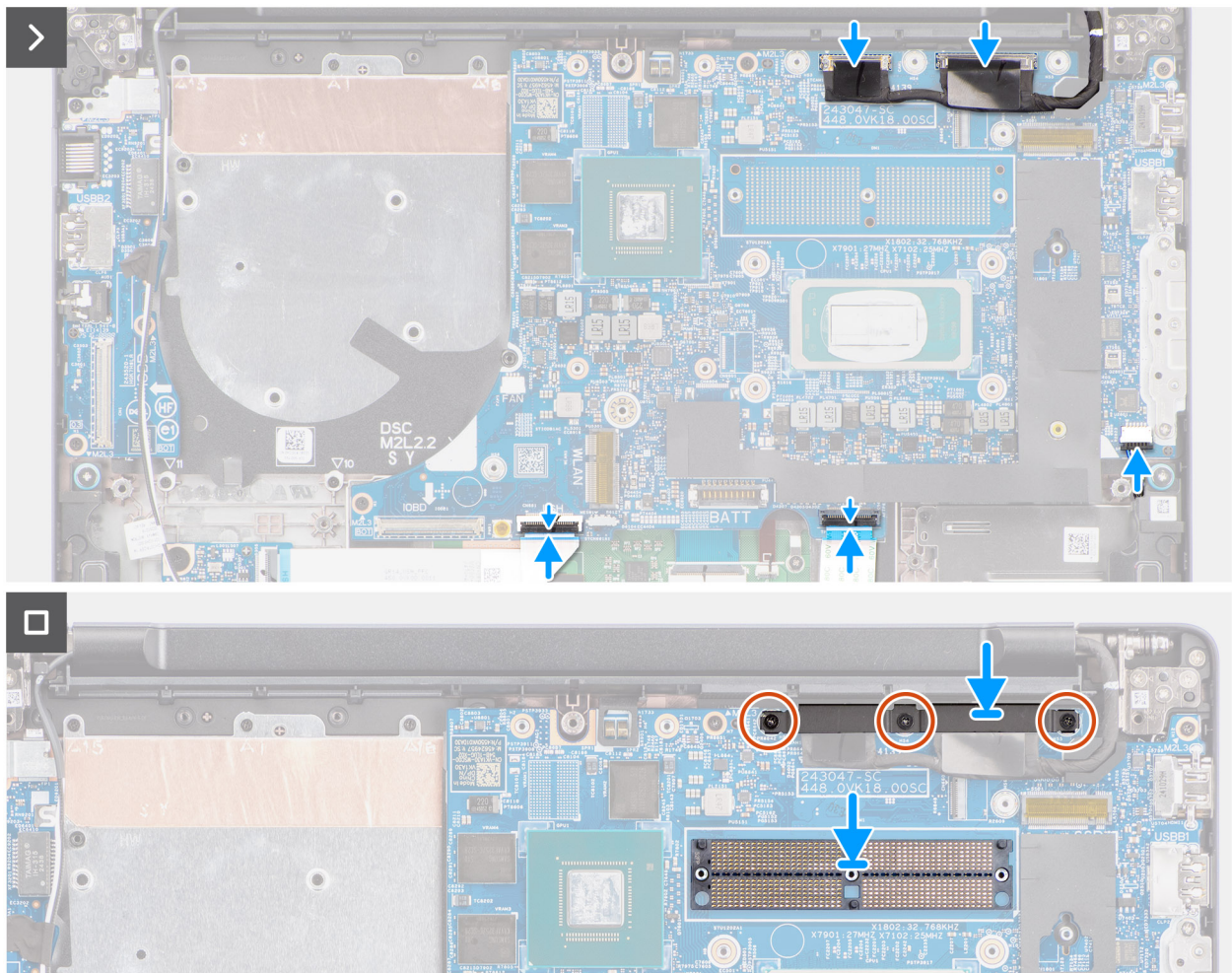
Abbildung 91. Einbauen der Systemplatine
