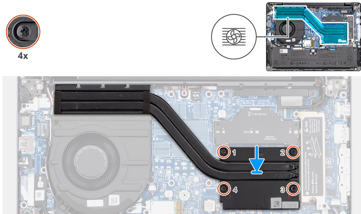
Abbildung 40. Installing the heat sink
