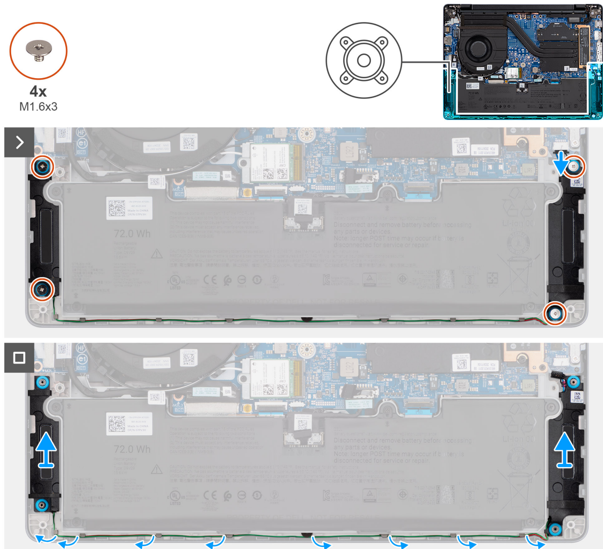
Abbildung 28. Removing the speakers
