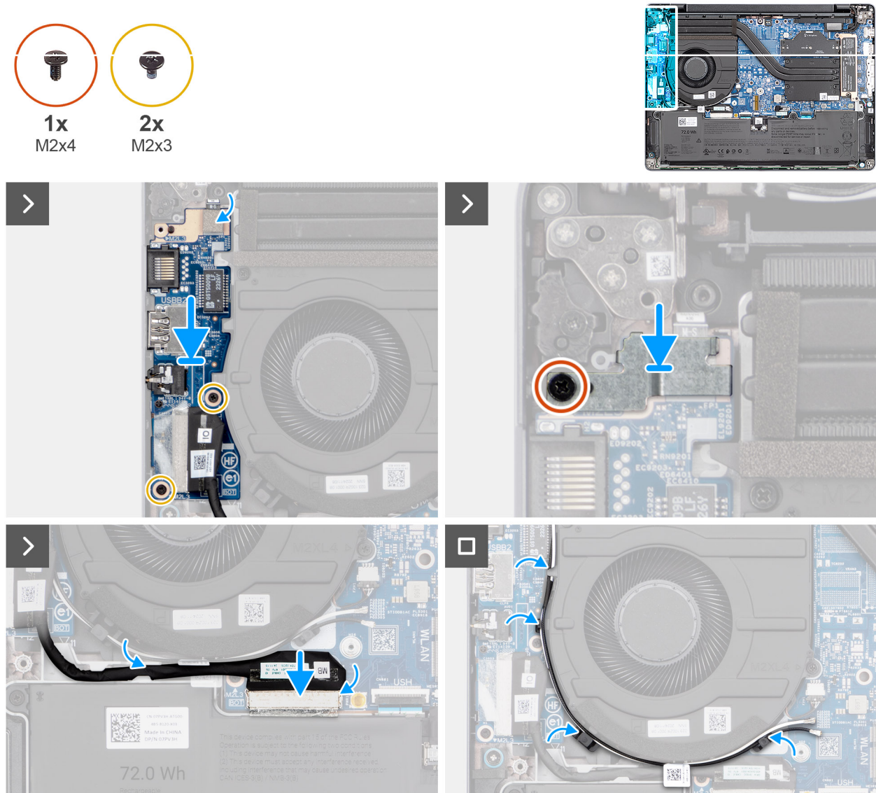
Abbildung 44. Installieren der I/O-Platine
