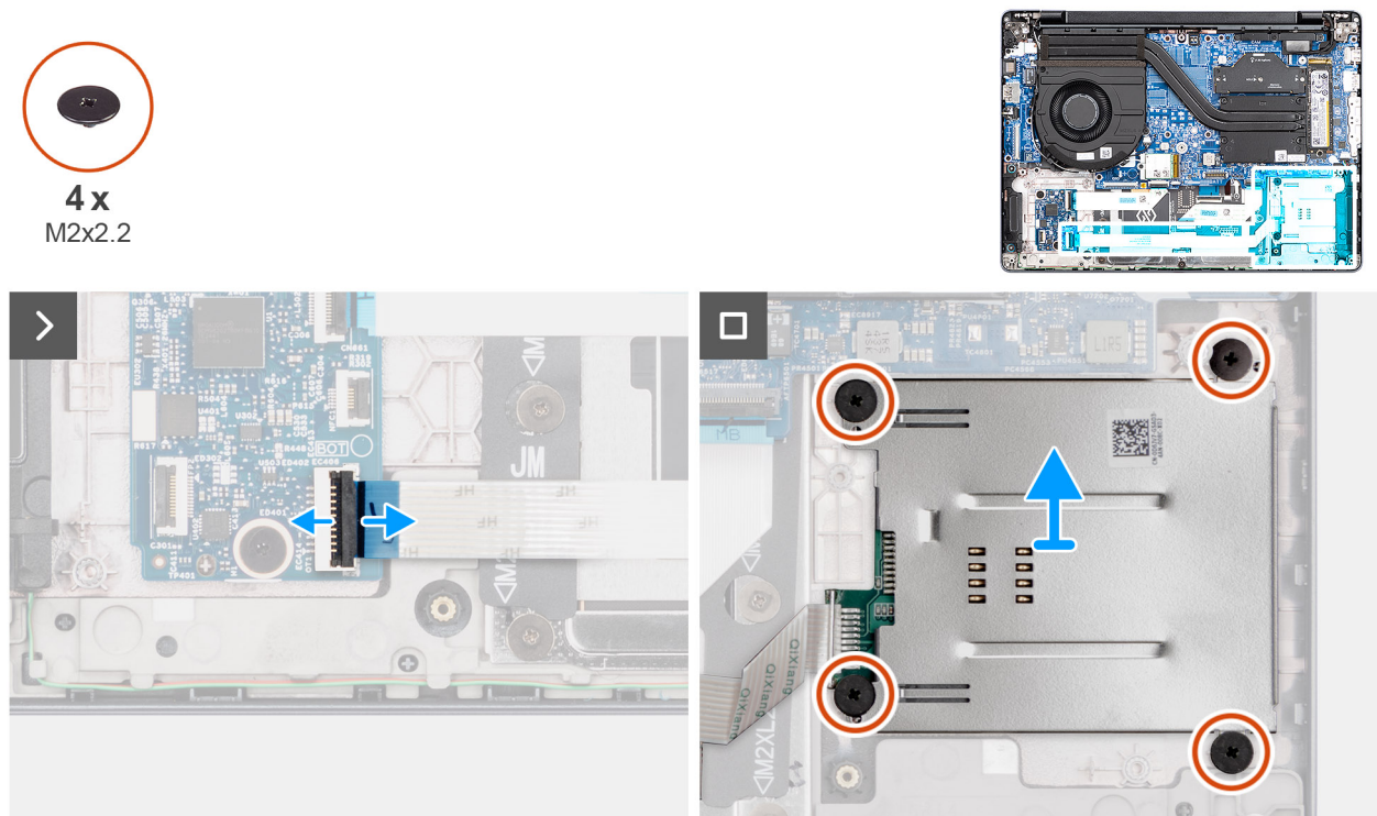
Abbildung 37. Entfernen des Smartcardlesegeräts
