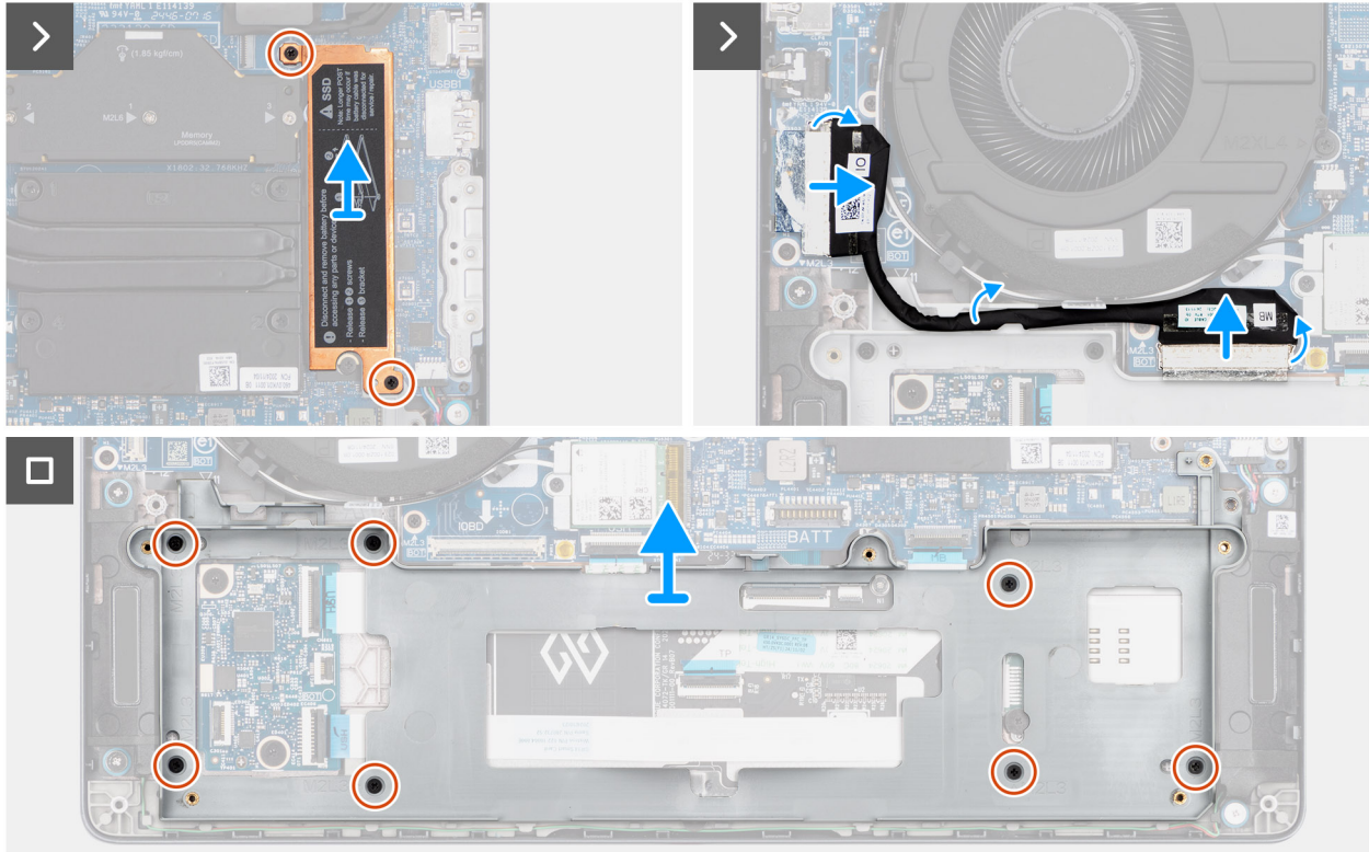
Abbildung 33. Entfernen des Akkurahmens
