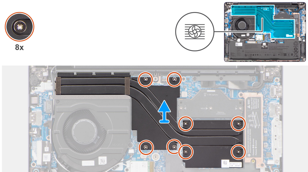
Abbildung 41. Kühlkörper entfernen
