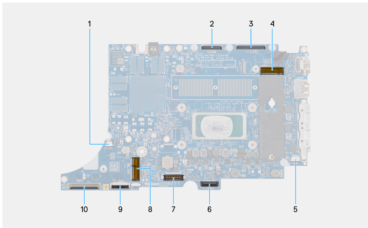
Abbildung 86. Anschlüsse auf der Hauptplatine
