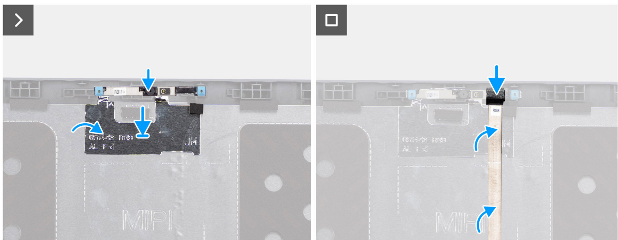
Abbildung 71. Installieren der Kamera
