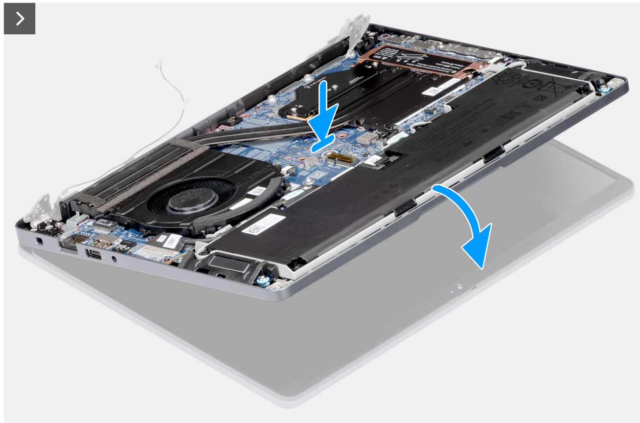
Abbildung 50. Einbauen der Bildschirmbaugruppe
