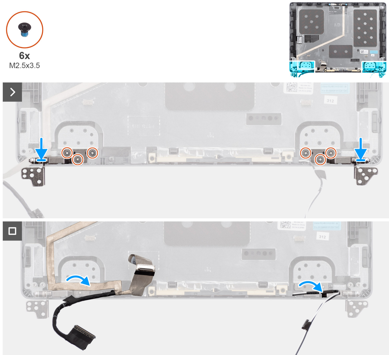
Abbildung 67. Installing the display hinges
