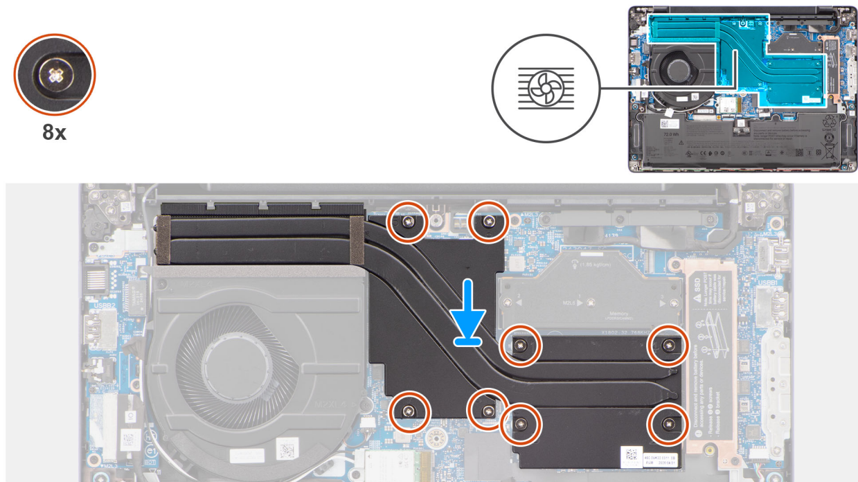
Abbildung 42. Einsetzen des Kühlkörpers
