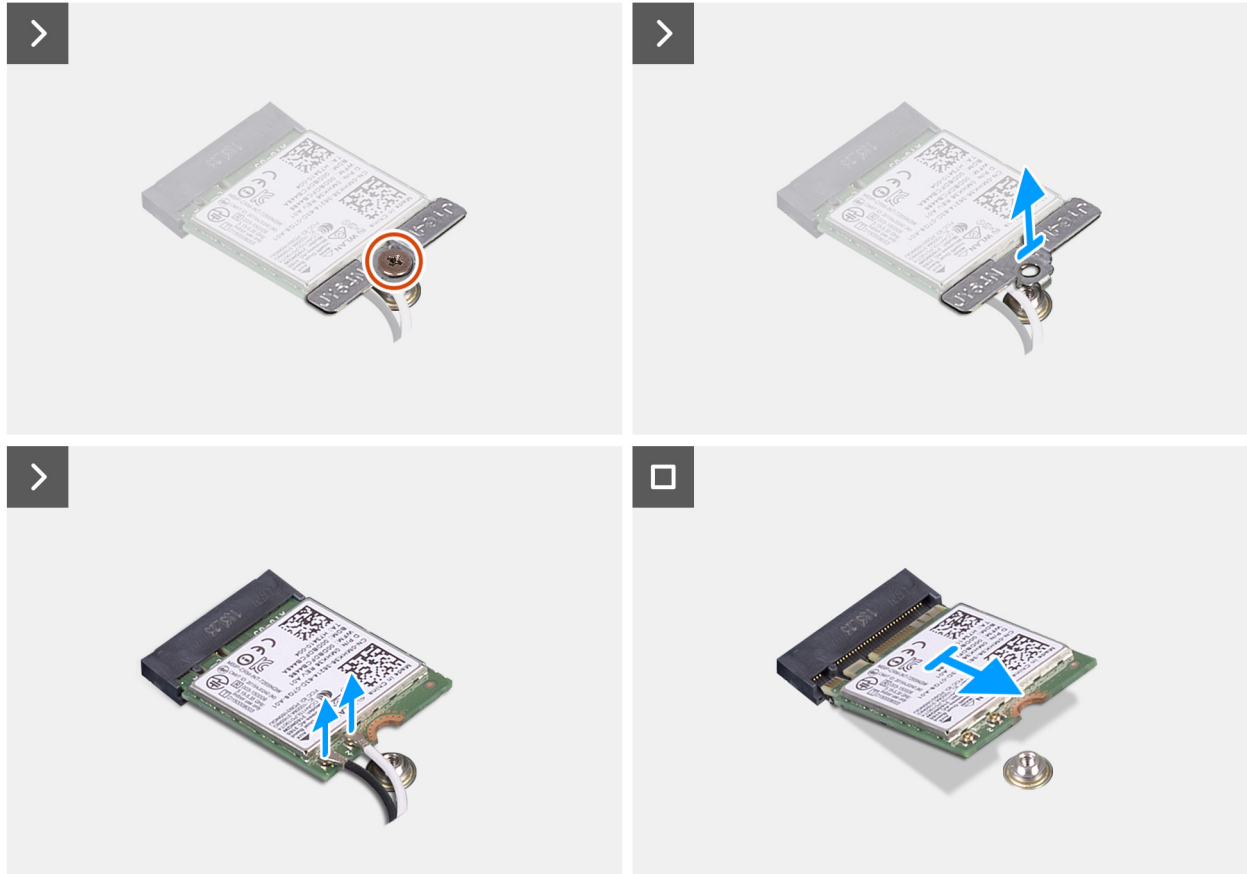
Abbildung 26. Entfernen der Wireless-Karte
