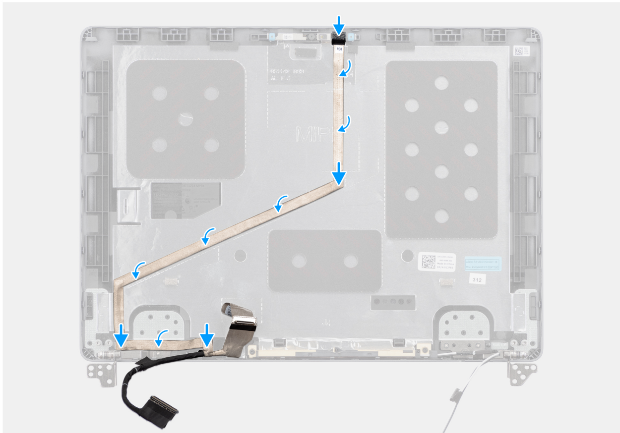
Abbildung 69. Installing the display cable
