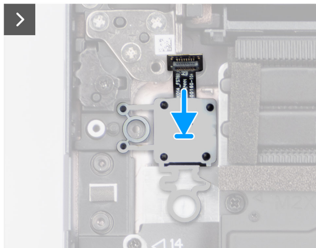
Abbildung 46. Installieren des Netzschalters
