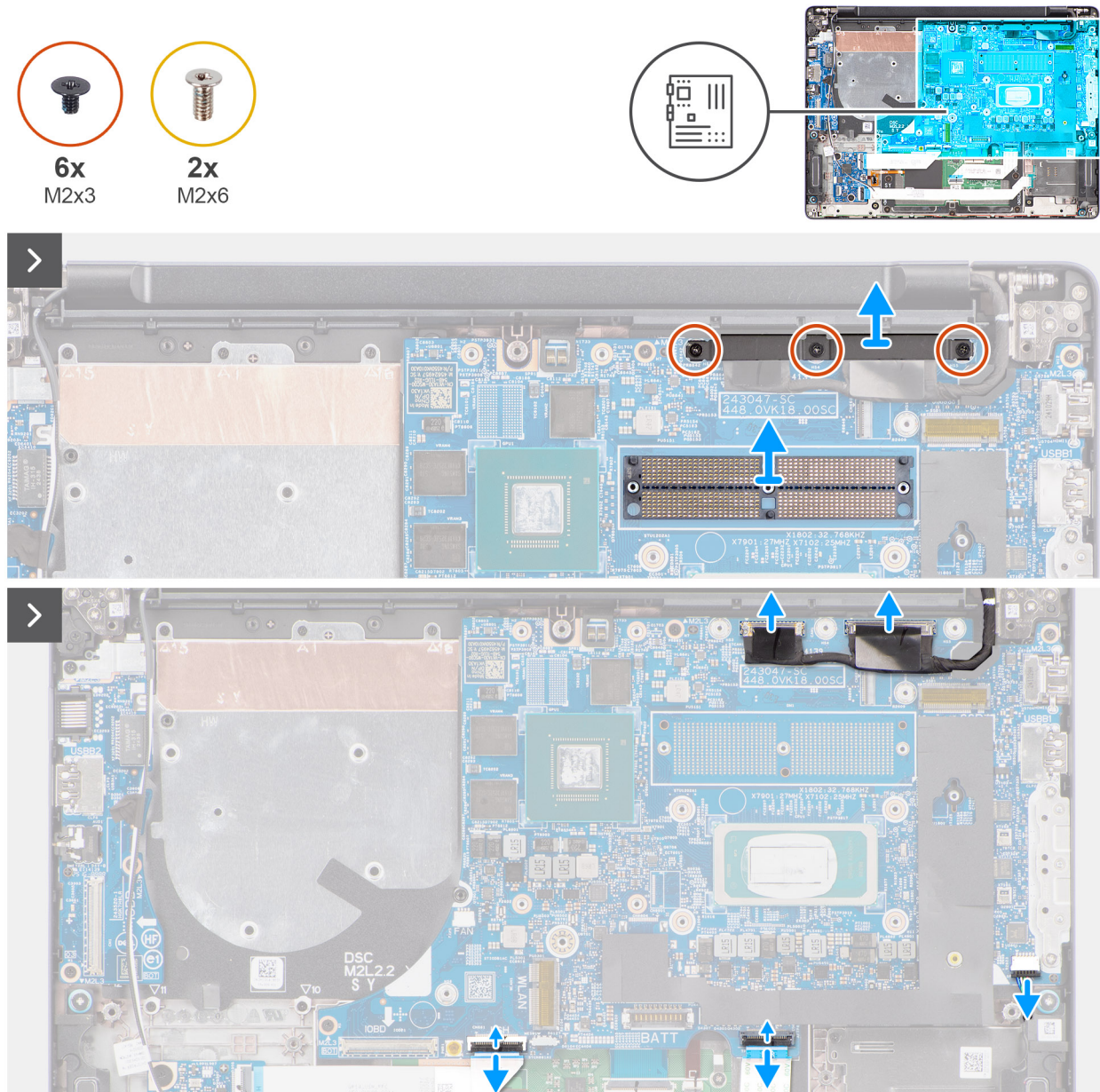
Abbildung 87. Entfernen der Systemplatine
