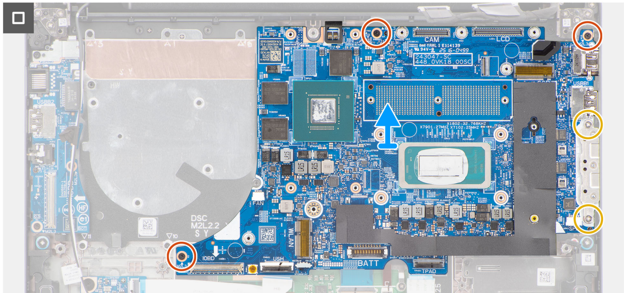
Abbildung 88. Entfernen der Systemplatine
