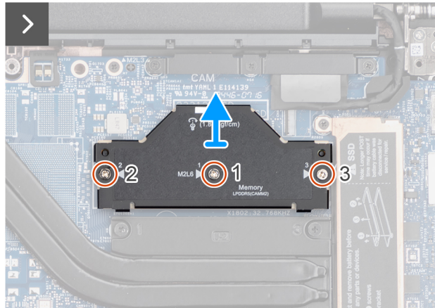
Abbildung 20. Entfernen des Arbeitsspeichermoduls
