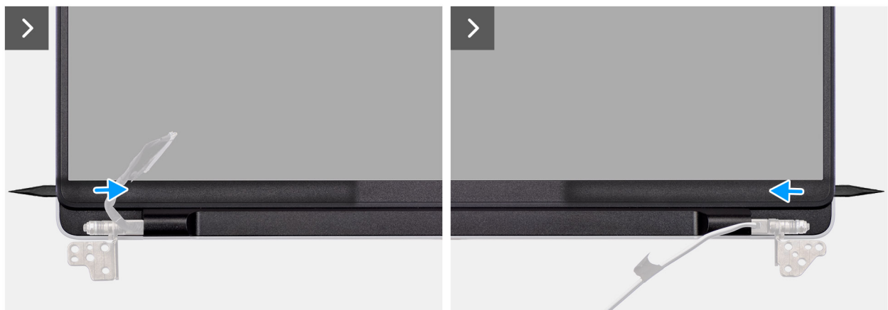
Abbildung 56. Removing the display bezel
