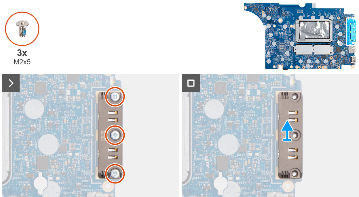
Abbildung 92. Removing the USB Type-C module
