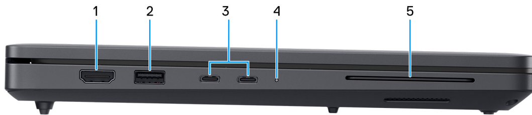
Abbildung 2. Linke Seitenansicht
