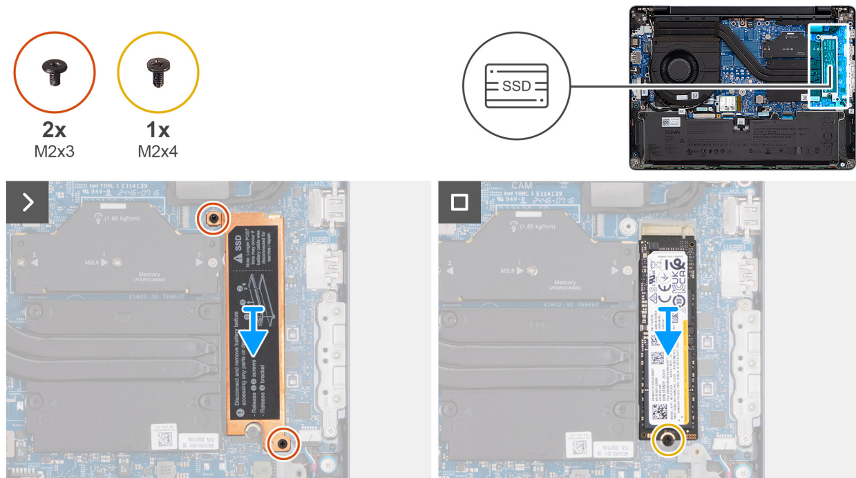
Abbildung 24. Removing the M.2 2280 solid state drive
