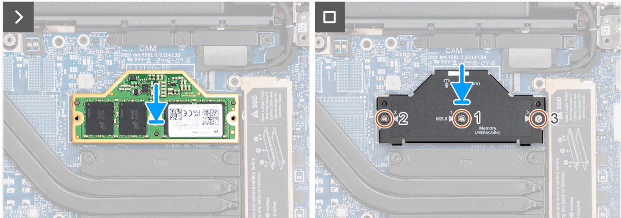
Abbildung 21. Einsetzen des Speichermoduls
