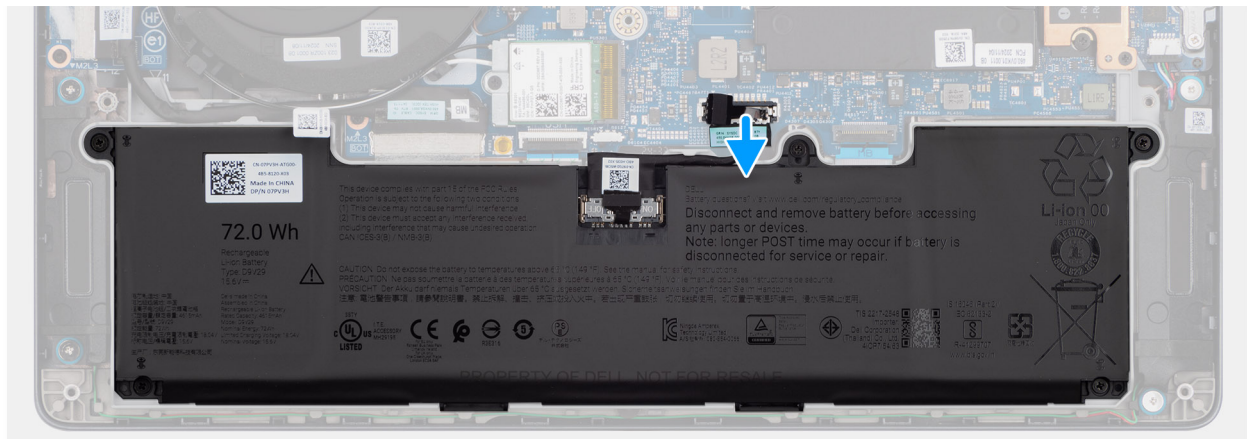
Abbildung 13. Entfernen des Akkukabels
