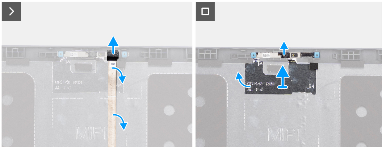
Abbildung 70. Entfernen der Kamera
