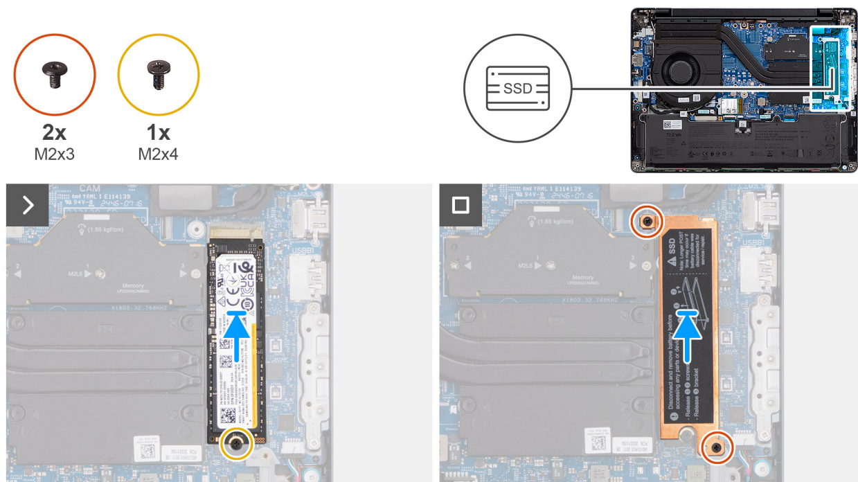
Abbildung 25. Installieren des M.2 2280-Solid-State-Laufwerks
