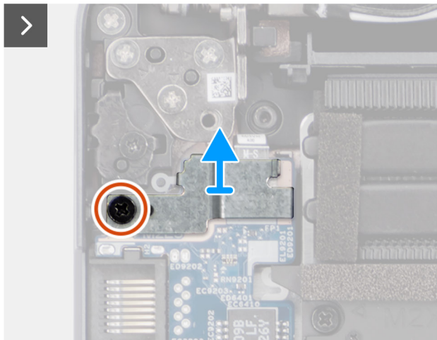
Abbildung 43. Entfernen der E/A-Platine
