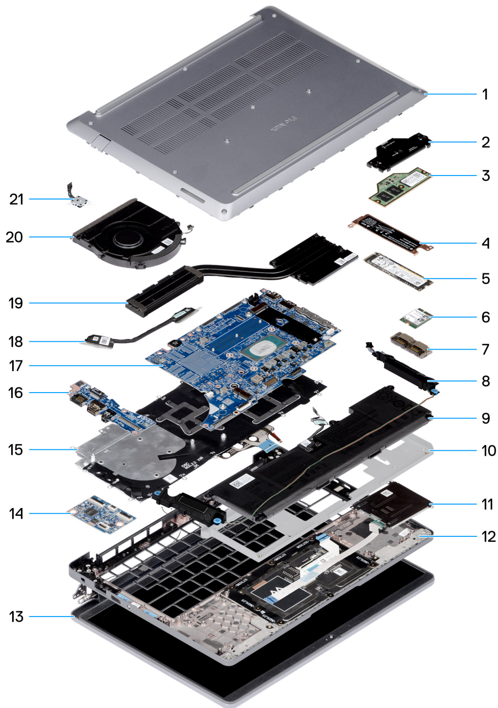
Abbildung 10. Hauptkomponenten Ihres Dell Pro Max 14 MC14250
