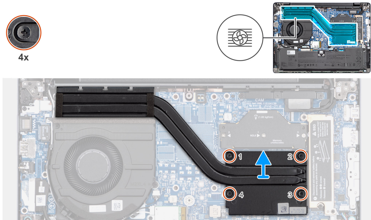
Abbildung 39. Kühlkörper entfernen
