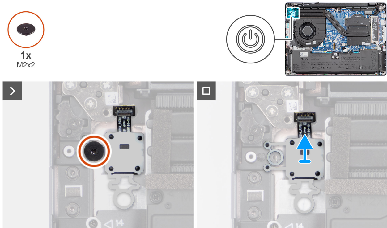
Abbildung 45. Removing the power button
