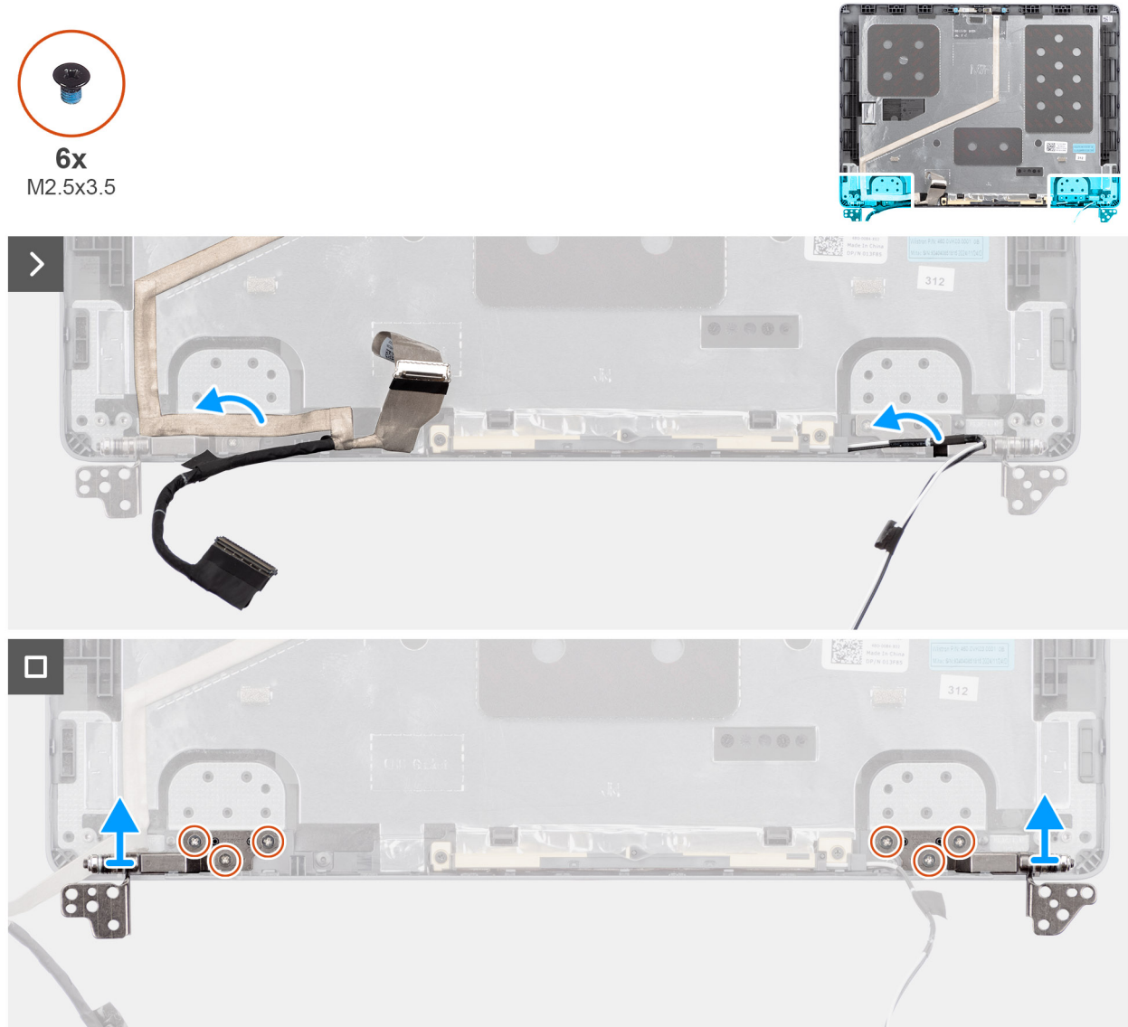
Abbildung 66. Removing the display hinges
