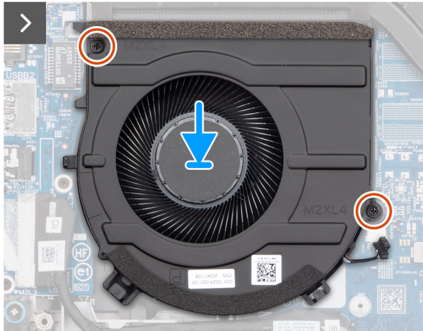
Abbildung 32. Installing the fan
