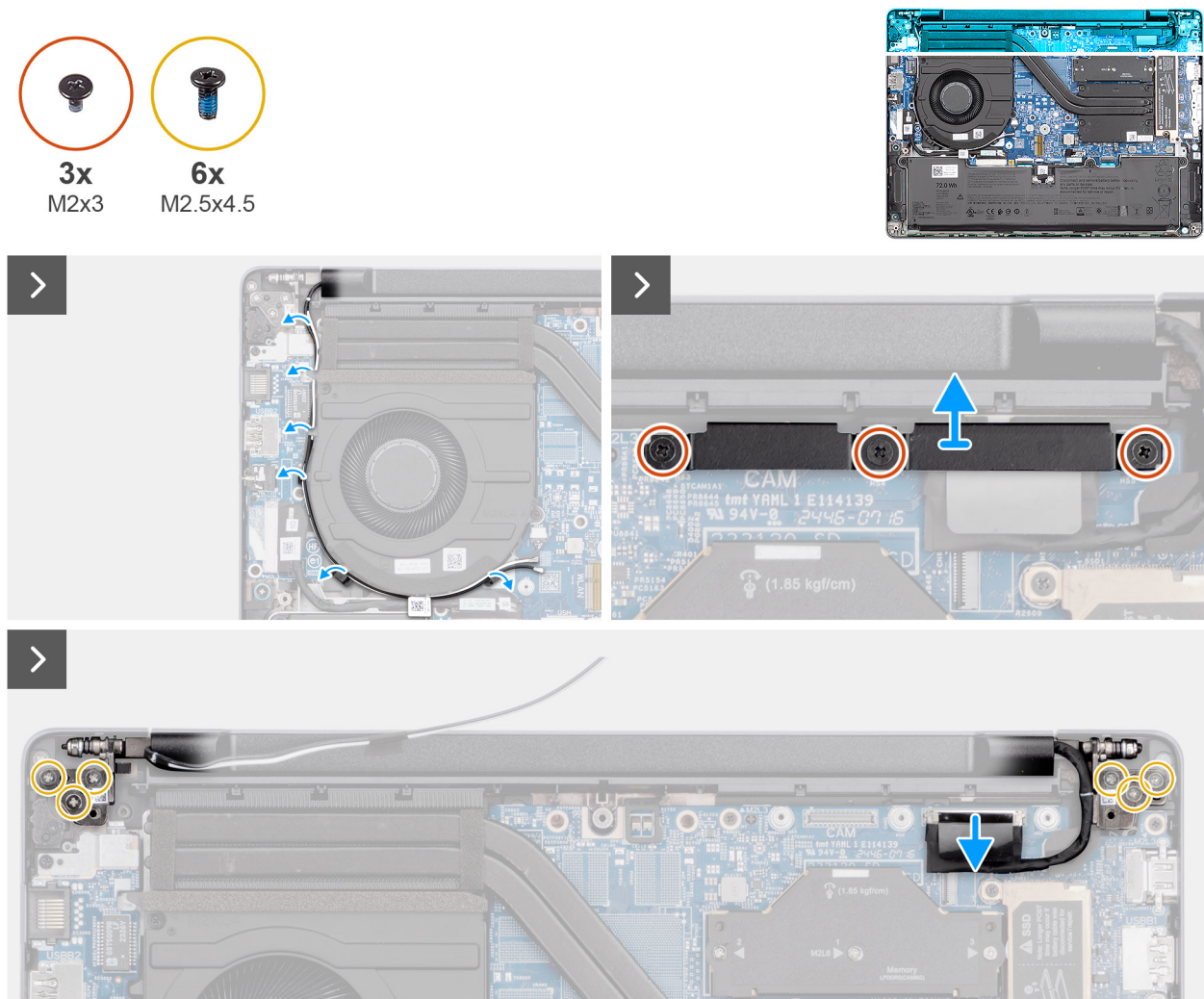
Abbildung 47. Entfernen der Bildschirmbaugruppe
