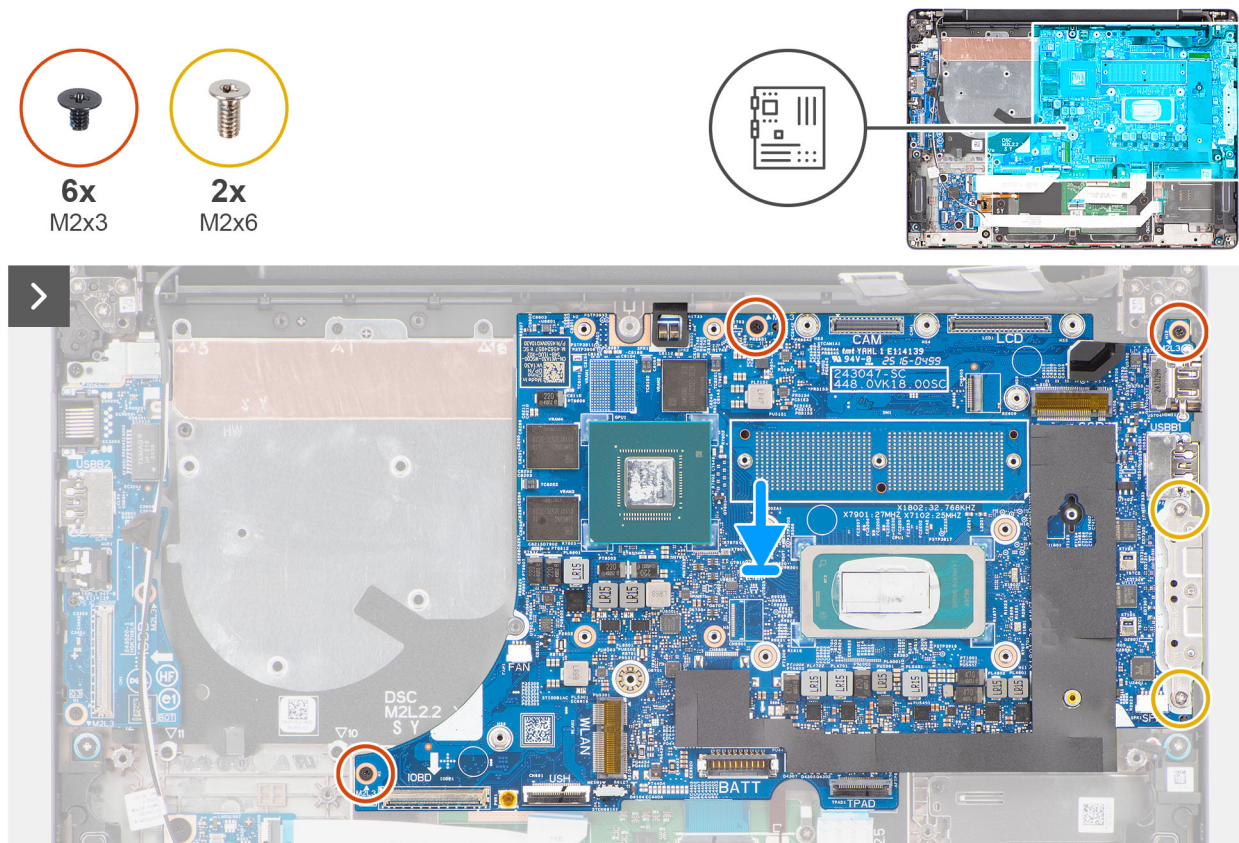
Abbildung 90. Einbauen der Systemplatine
