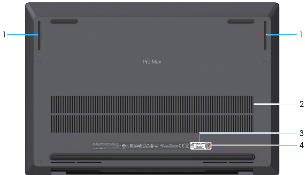
Abbildung 6. Untere Ansicht
