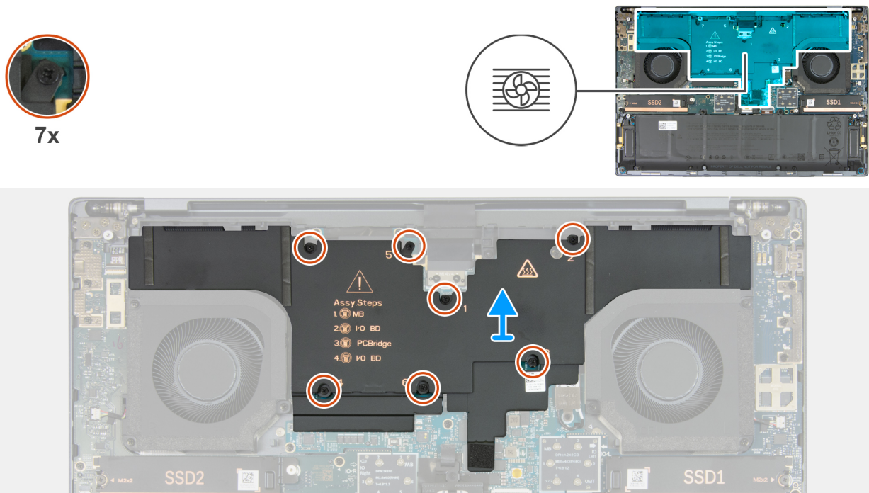
Abbildung 48. Kühlkörper entfernen
