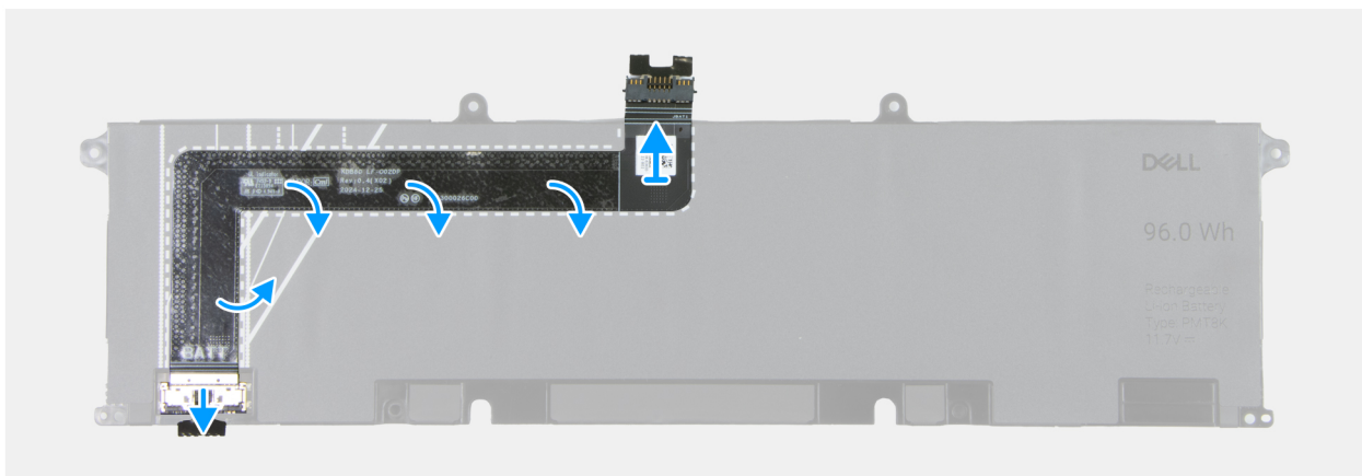
Abbildung 20. Entfernen des Akkukabels
