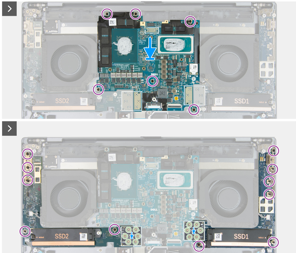
Abbildung 68. Einbauen der Hauptplatine (separate Grafikkarte)
