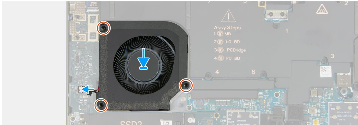
Abbildung 33. Installieren des rechten Lüfters
