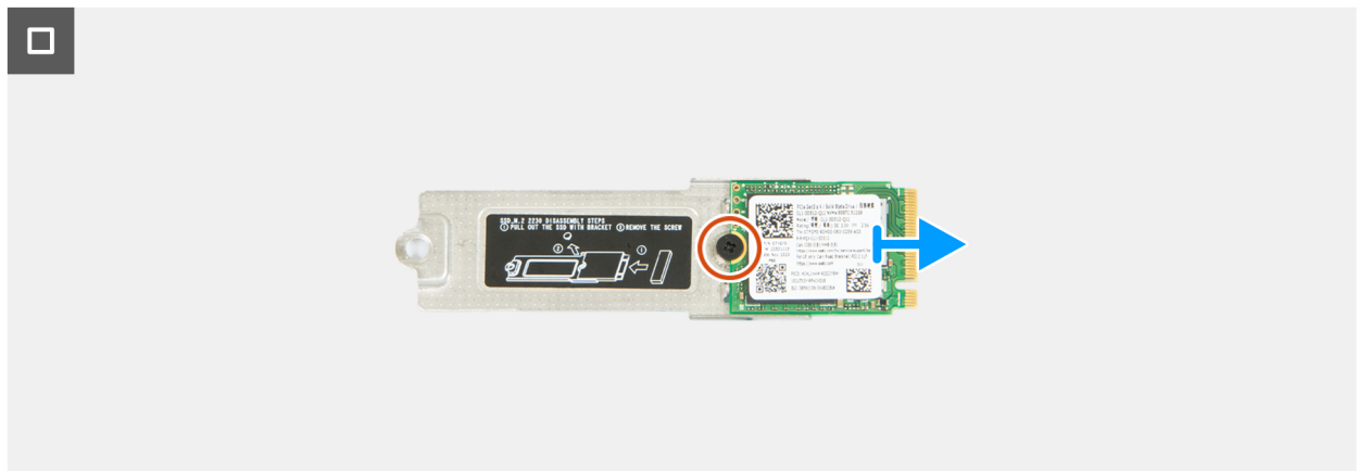
Abbildung 26. Entfernen des M.2 2230-Solid-State-Laufwerks (SSD1)
