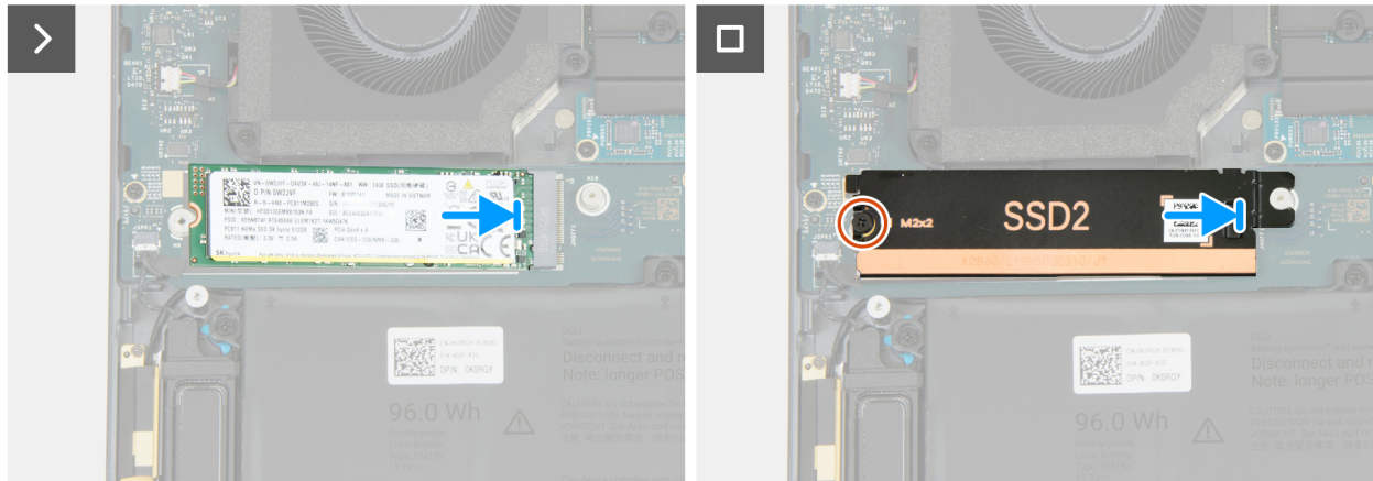
Abbildung 25. Einbauen des M.2 2280-Solid-State-Laufwerks (SSD2)
