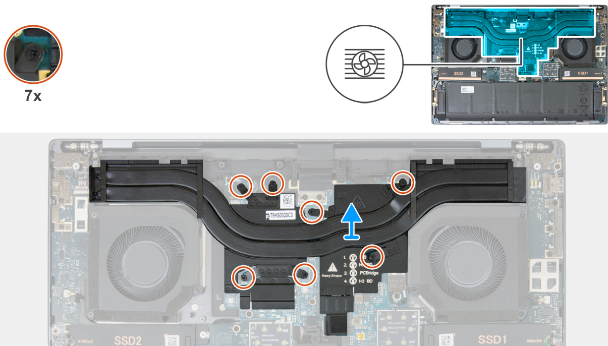
Abbildung 46. Kühlkörper entfernen
