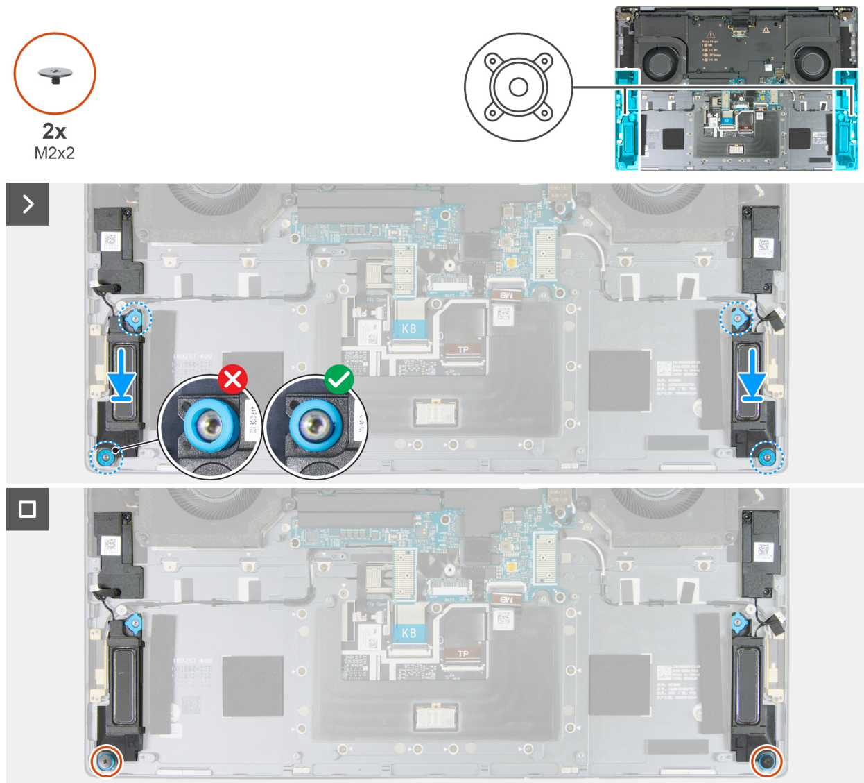
Abbildung 75. Installieren der Lautsprecher
